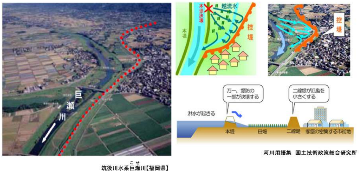
巨瀬川二線堤(控え堤) (福岡県久留米市)
