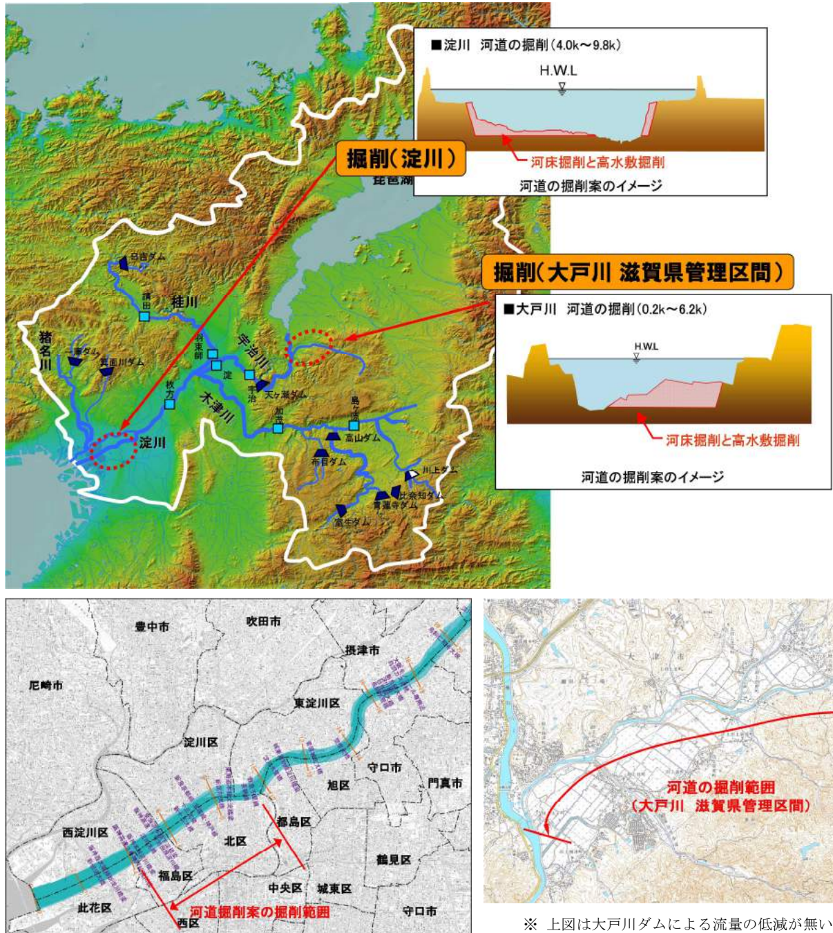
図 4.2-10 河道掘削区間位置図と掘削のイメージ図
