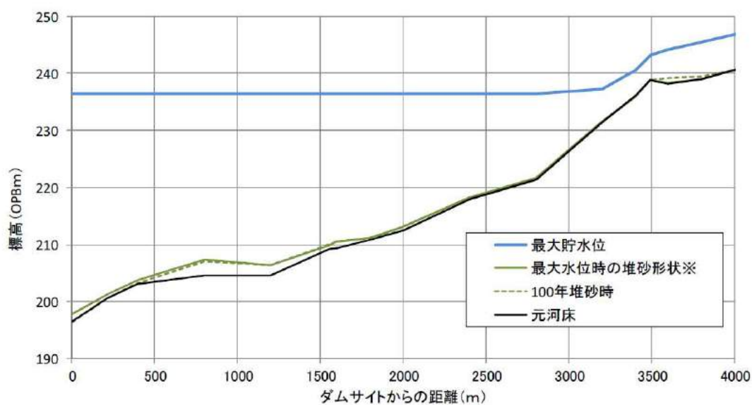
図 4.1-4 ダム貯水池の推定堆砂形状
