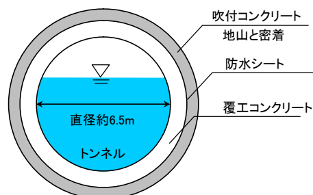
放水路(海ルート)イメージ (200m³/s規模のトンネル×3条)
