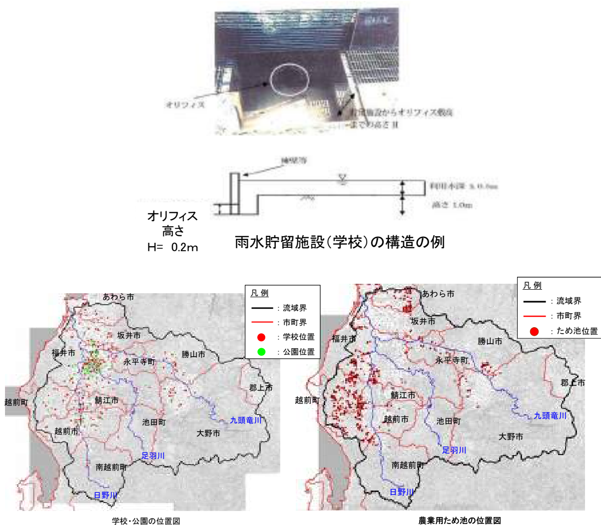
図 4-18 雨水貯留施設のイメージ
