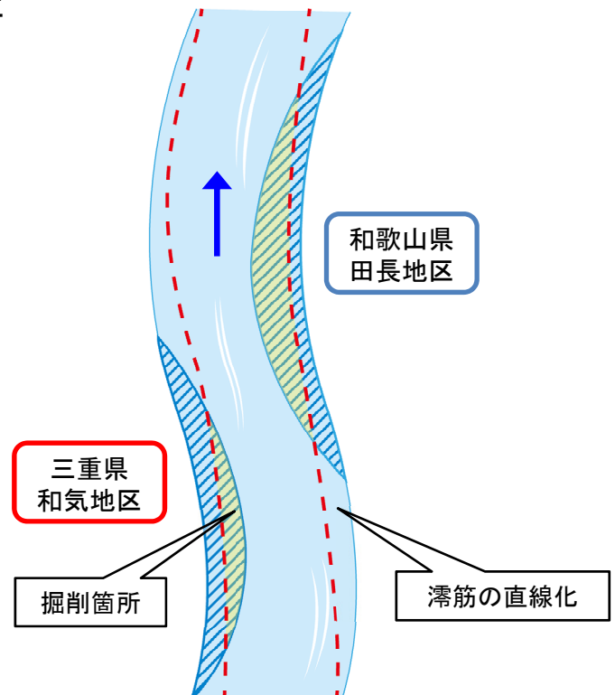
滞筋の直線化を踏まえた掘削計画のイメージ図
