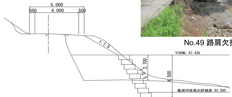
横断面図
