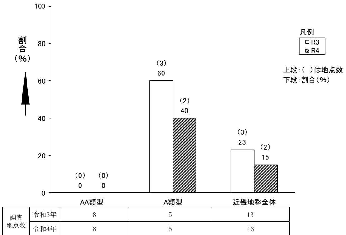
図-1.2 湖沼類型指定地点における類型別環境基準の満足状況 (令和3年、令和4年) (COD75%値)
