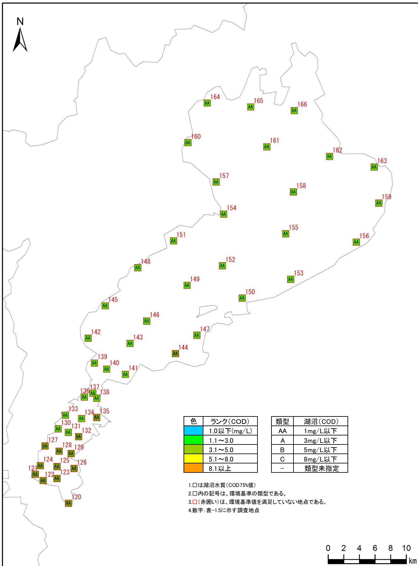
図-1.8 琵琶湖における水質状況(COD75%値)
