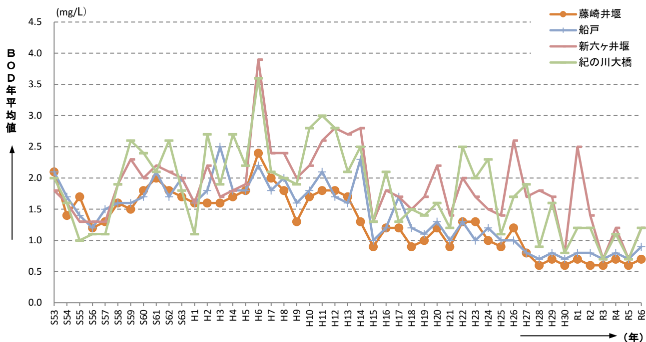
図－1.11 紀の川（下流）の水質経年変化（BOD年平均値）
