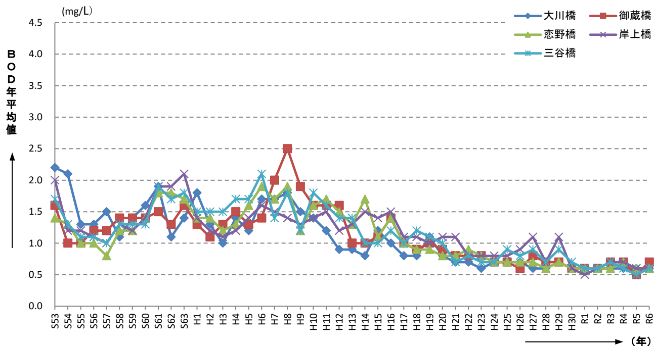
図－1.10 紀の川（上流）の水質経年変化（BOD年平均値）
