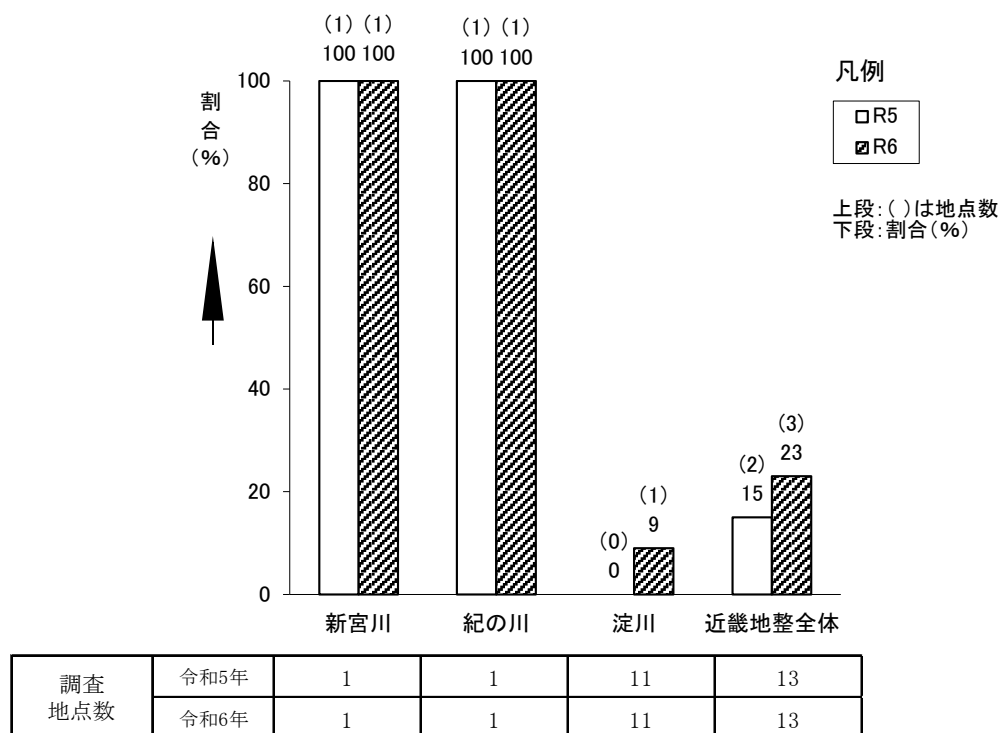
図－1.4 湖沼類型指定地点における水系別環境基準の満足状況 (令和5年、令和6年) (COD75%値)
