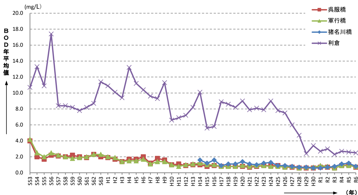
図-1.22 猪名川の水質経年変化（BOD年平均值）
