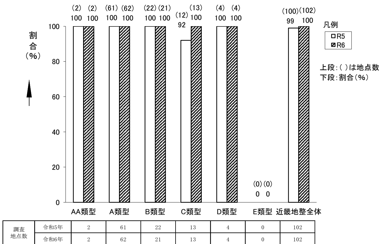
図－1.1 河川類型指定地点における類型別環境基準の満足状況 (令和5年、令和6年) (BOD75%値)
