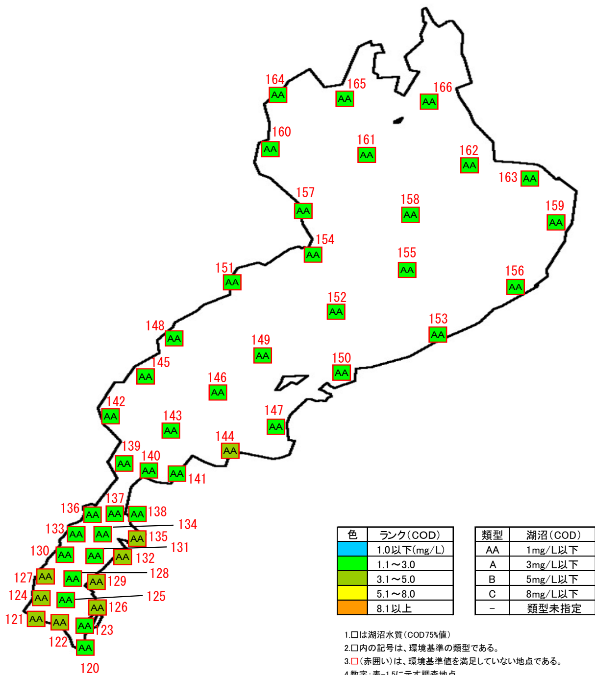
図-1.8 琵琶湖における水質状況 (COD75%値)
