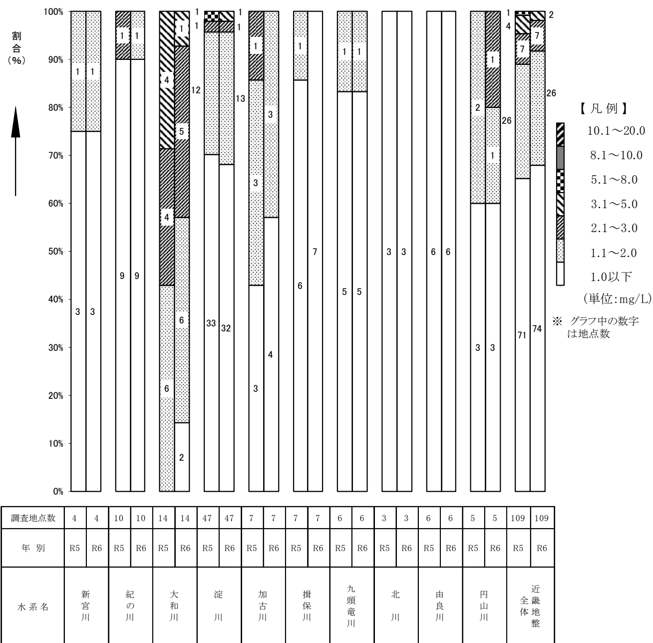
図－1.6 水系別BOD75%値のランク別割合（109 地点）
