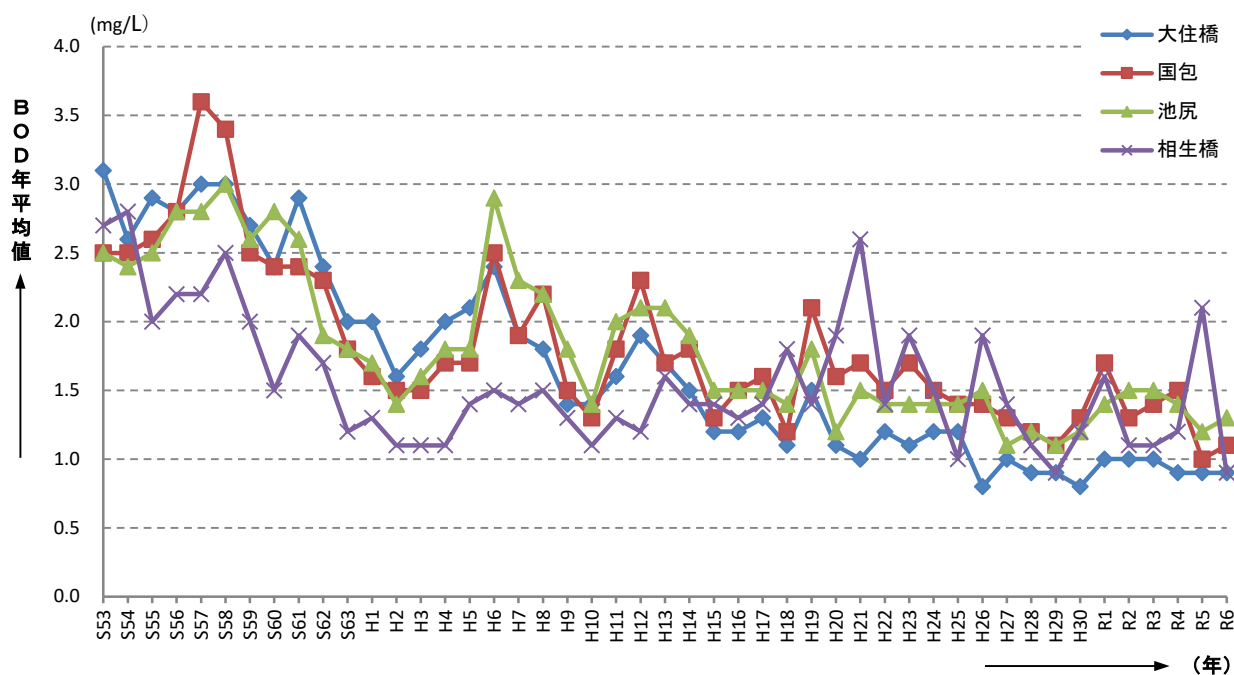
図-1.23 加古川の水質経年変化（BOD年平均值）
