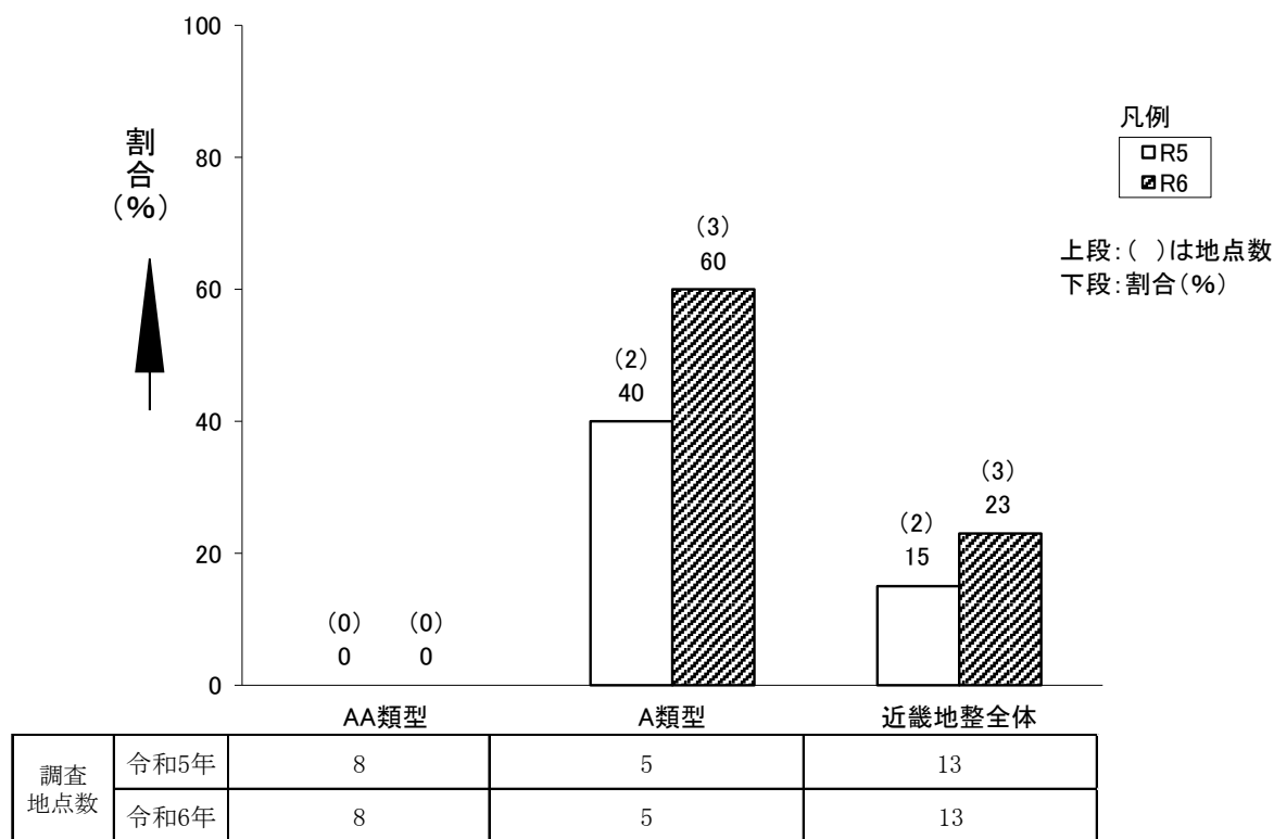
図－1.2 湖沼類型指定地点における類型別環境基準の満足状況 (令和5年、令和6年) (COD75%値)
