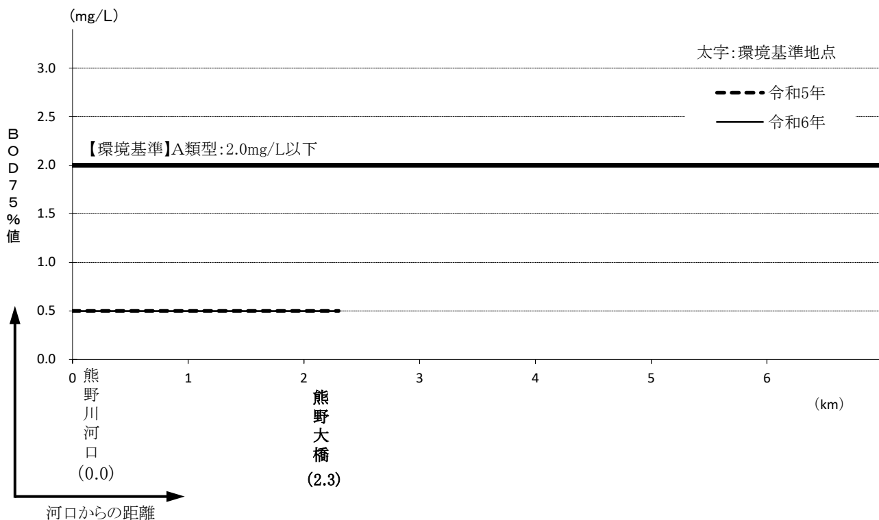
図－1.31 熊野川の水質縦断面図（BOD75%値）
