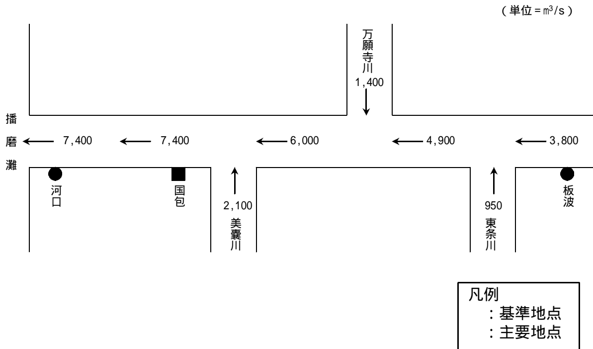
加古川計画高水流量図
