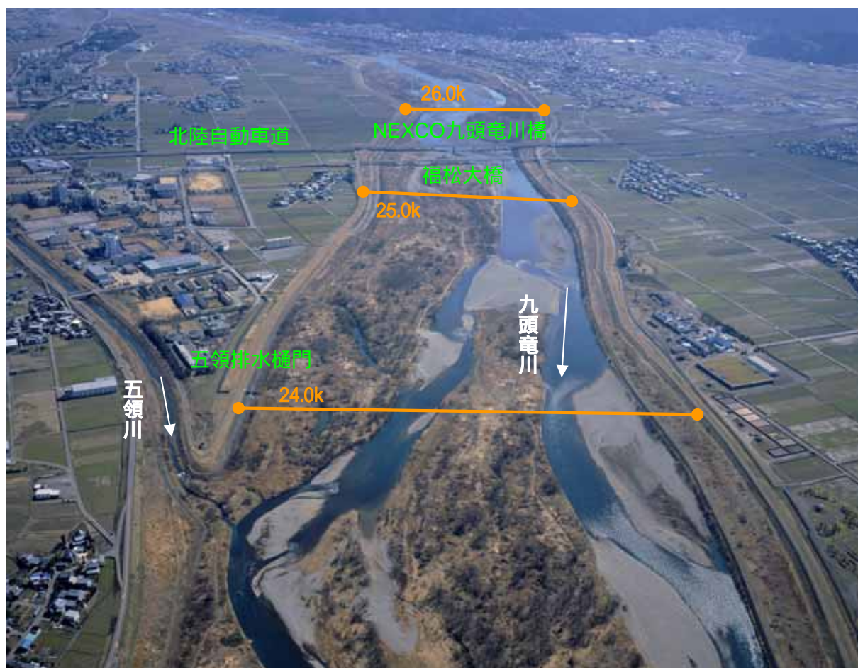
24.0k付近から上流部を望む(平成20年3月撮影)
