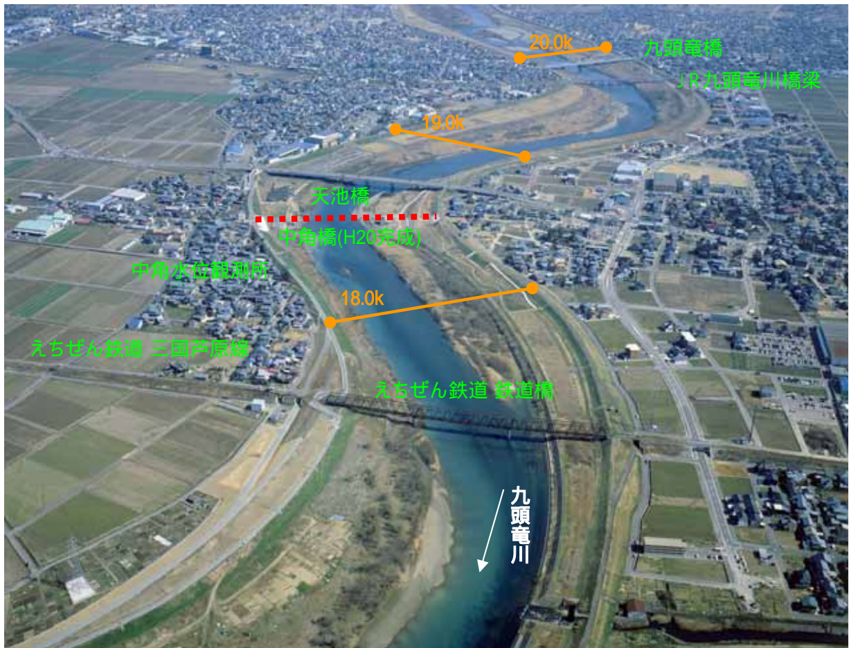
18.0k付近から上流部を望む(平成19年2月撮影)
