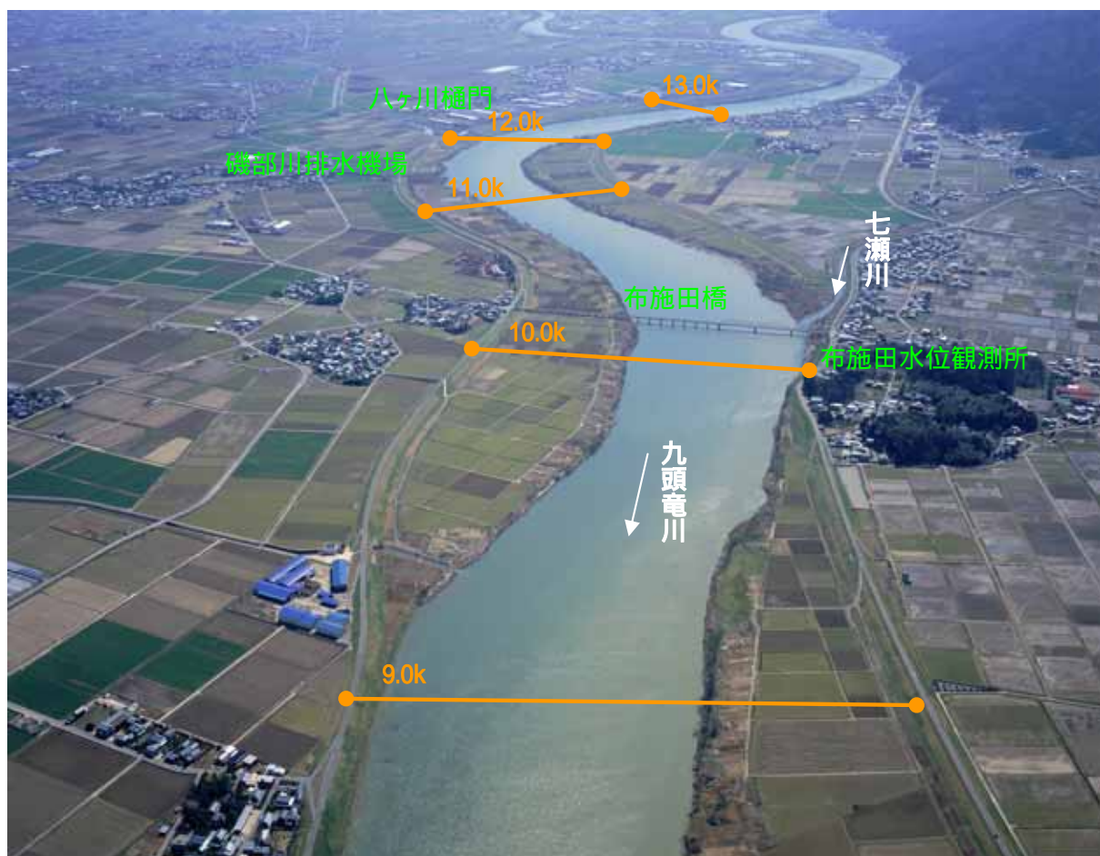
9.0k付近から上流部を望む(平成20年3月撮影)
