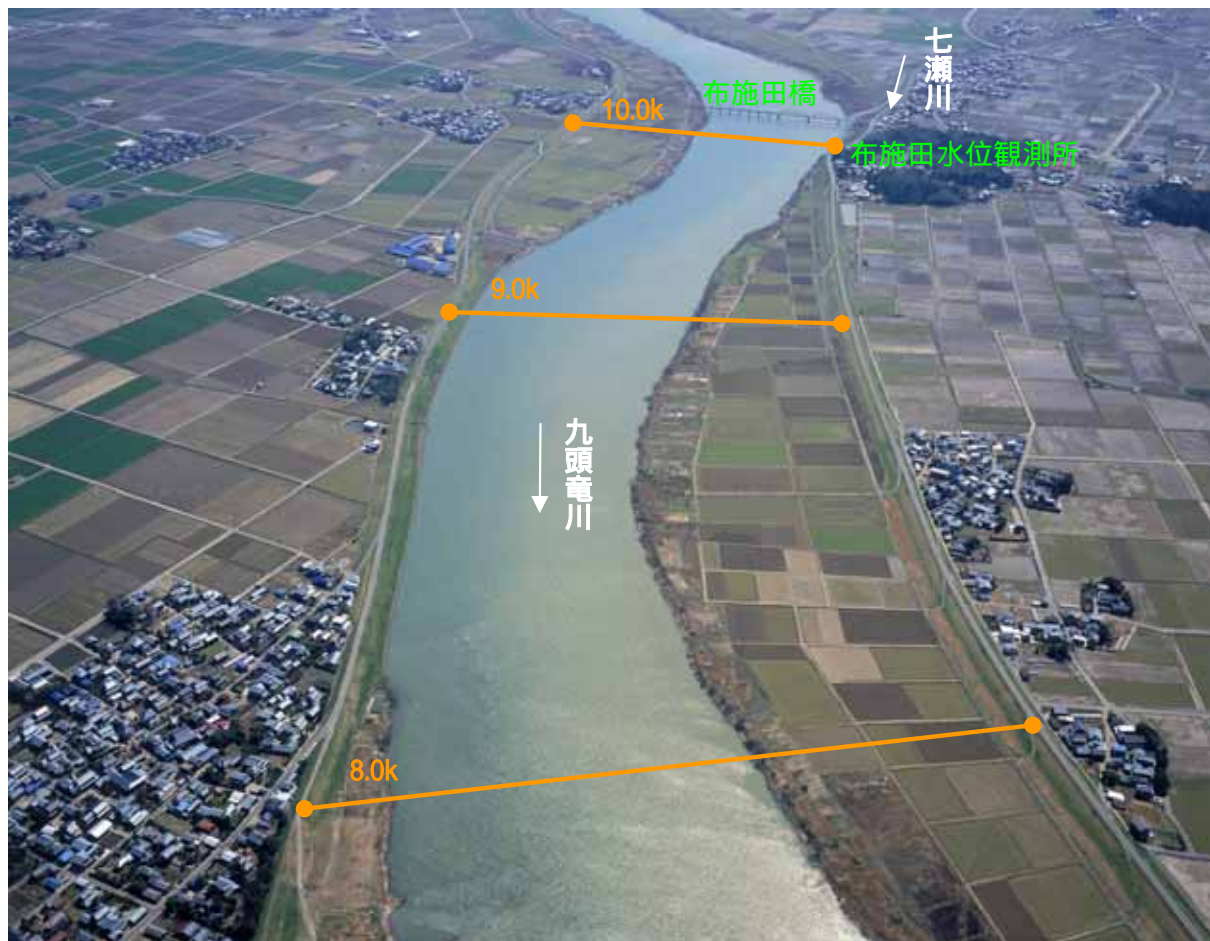
8.0k付近から上流部を望む(平成20年3月撮影)
