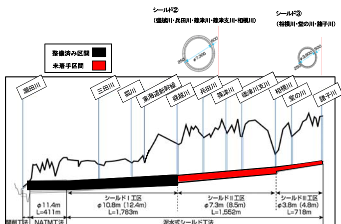
図 4.3.2-26 大津放水路断面図
