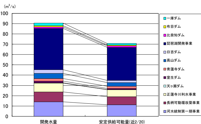
図 3.4-5 淀川水系における安定供給可能量
