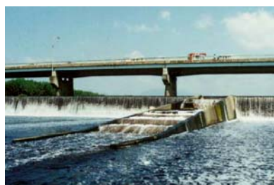
写真 4.2.3-8 桂川1号井堰
