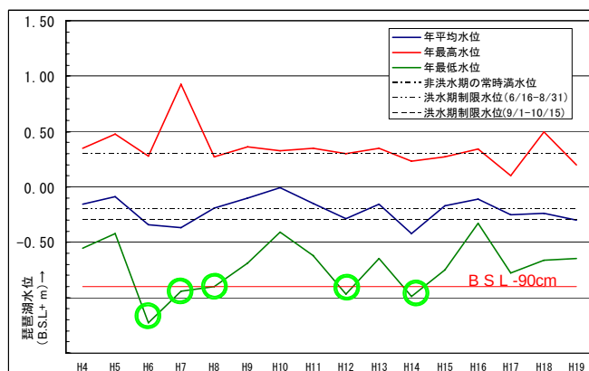
図 3.4-6 琵琶湖年水位グラフ
