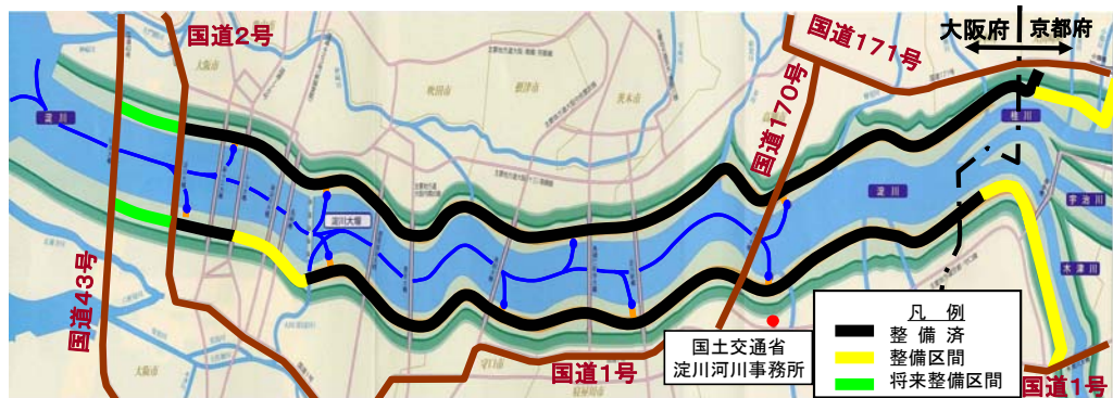
図 4.3.4-1 緊急用河川敷道路整備区間
