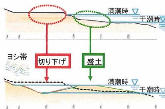
図 4.2.3-1 干潟造成イメージ
