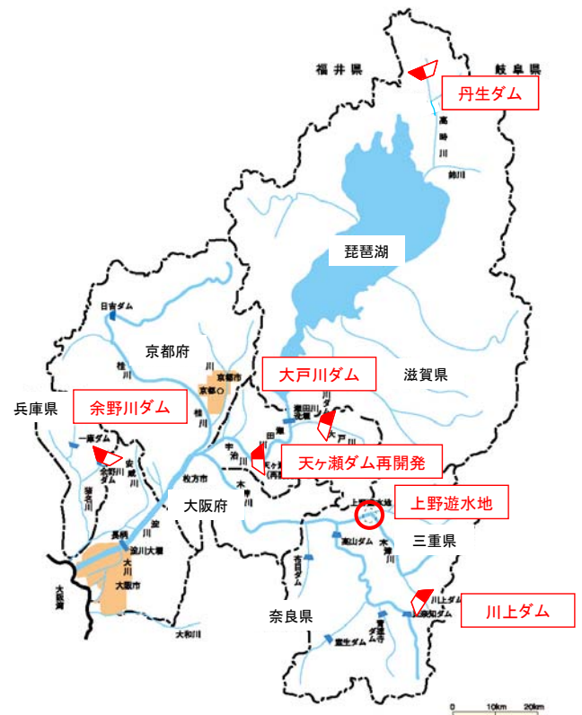
図 4.3.2-16 ダム等の位置図
