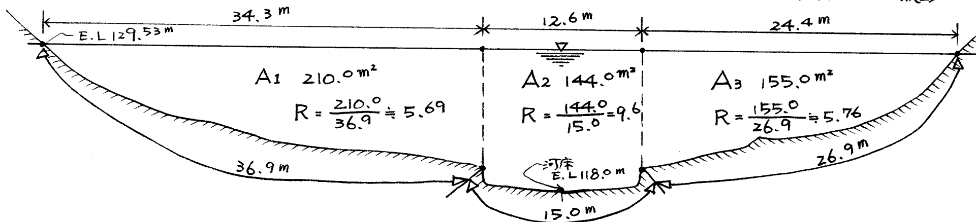
流体横断面図(岩倉峽最狹窄部)
