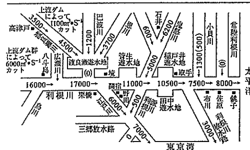
図2 利根川の高水流量配分図
