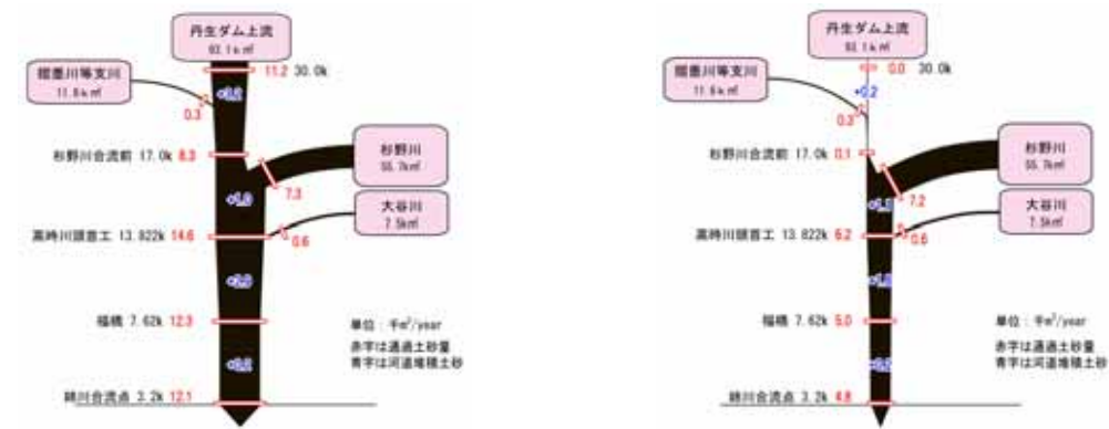
図 5.1.7 丹生ダムなし（全流砂）
