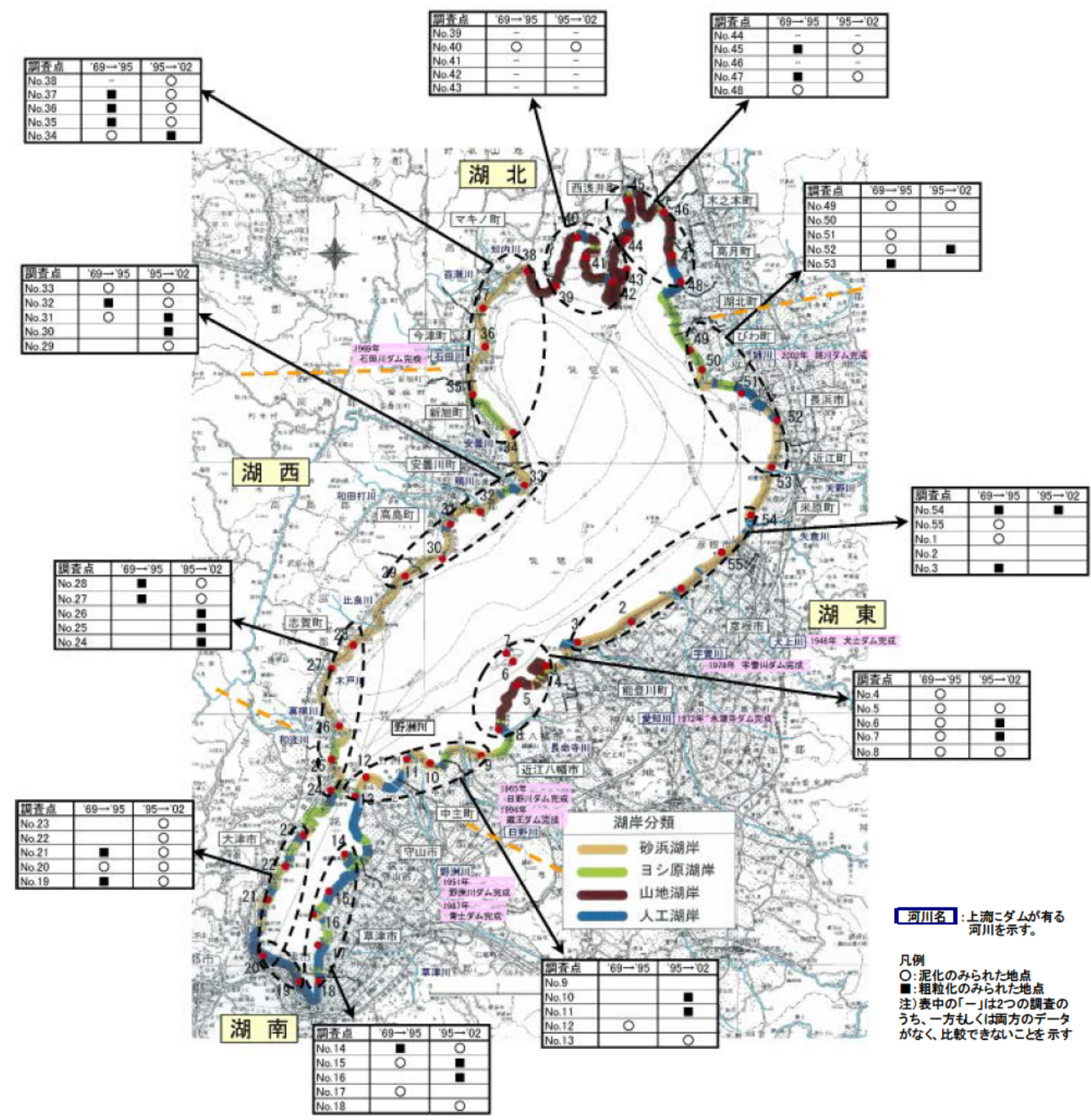
図 6.1.3 泥化・粗粒化の傾向
