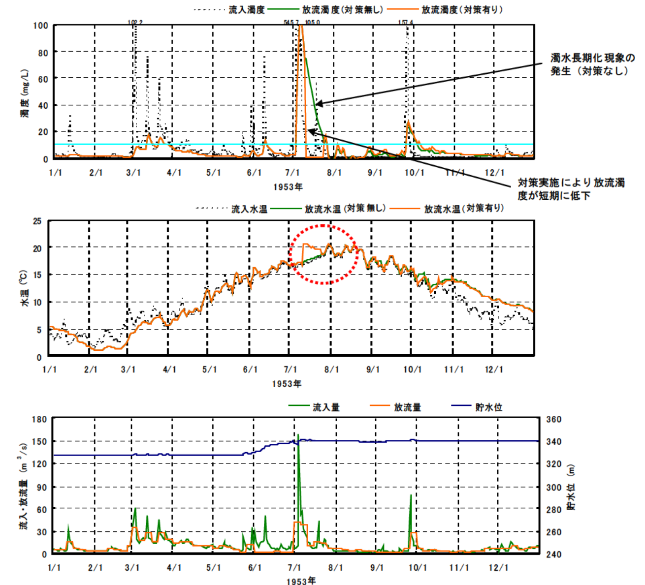
図 4.1.5 既往最大出水時における対策実施による放流濁度の変化
