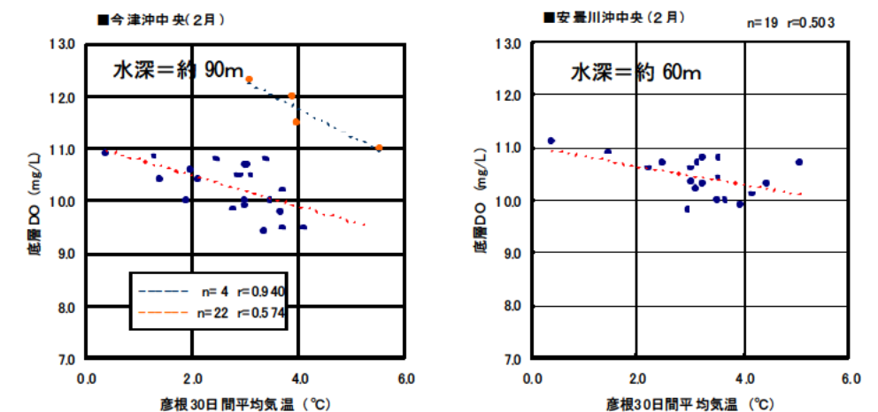
図 3.1.5 気温と琵琶湖深層部における溶存酸素の関係
