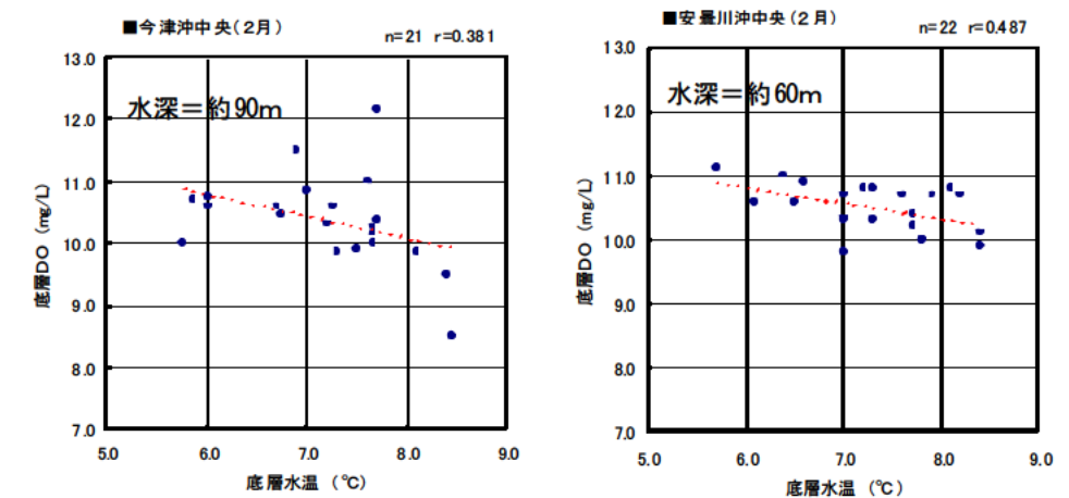
図 3.1.4 琵琶湖深層部における水温と溶存酸素の関係
