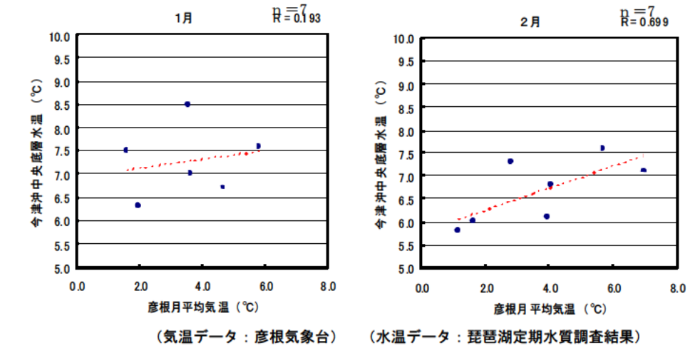
図 3.1.3 琵琶湖完全循環期（1～2月）における月平均気温と各地点底層水温の関係（その2）
