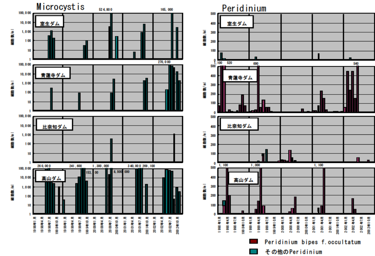
図 4.1.16 室生・青蓮寺・比奈知ダムー高山ダムの Microcystis、Peridinium 発生状況
