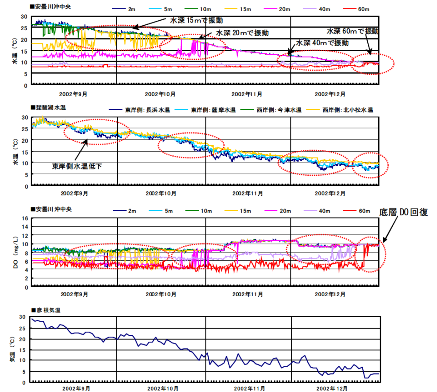
図 3.1.1 琵琶湖冷却期における水温・DOの動向（2002年9月～12月の例）
