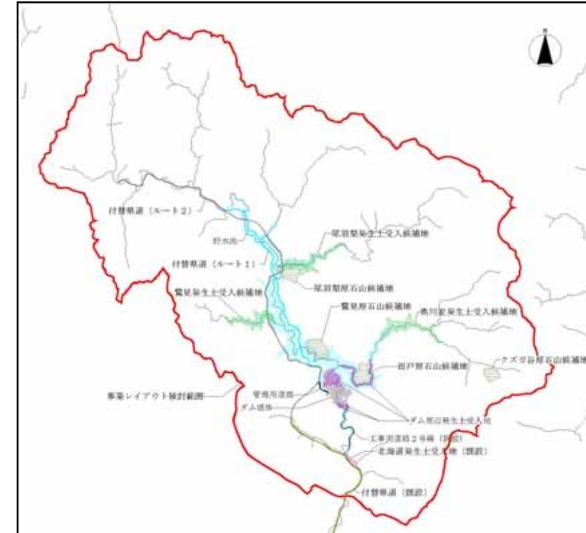
図ー1 丹生ダム事業レイアウト検討案
