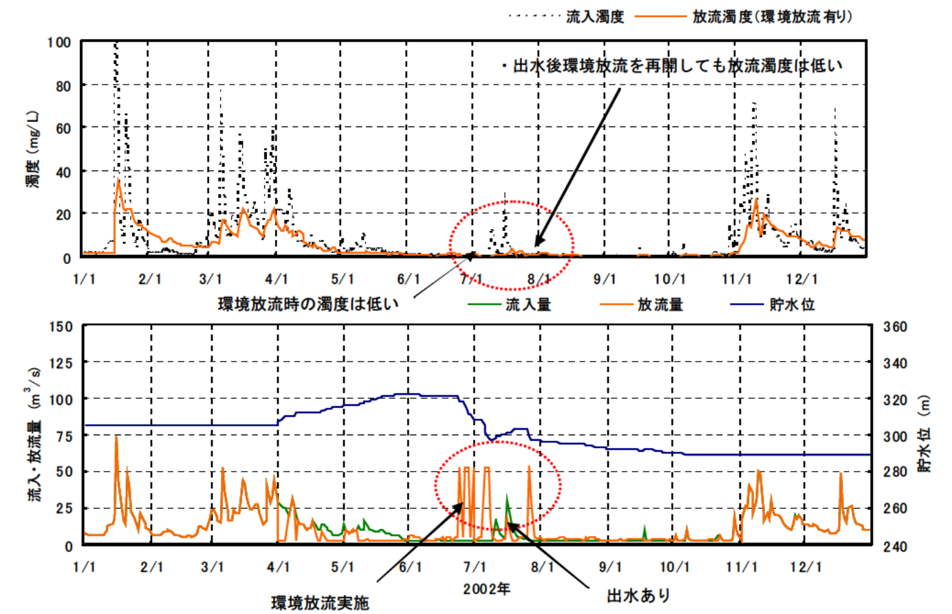
図 4.1.4 丹生ダムにおける環境放流を実施した場合の放流濁度の予測結果（2002 年）
