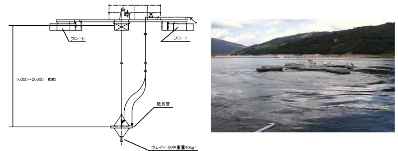
図 4.1.2 曝気装置概要図および曝気装置運転の様子（草木ダム）
