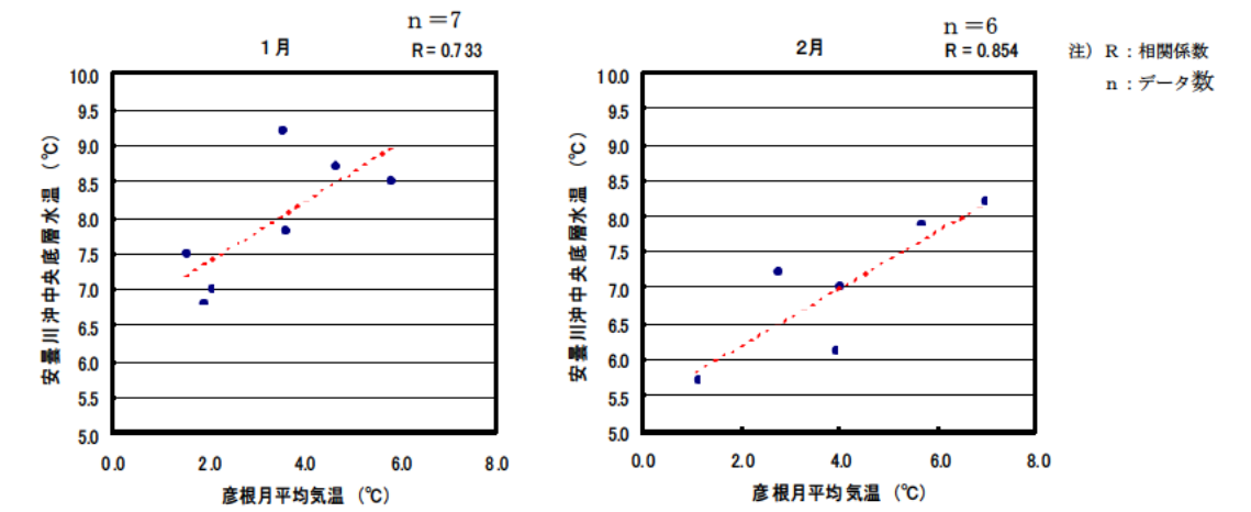
図 3.1.2 琵琶湖完全循環期（1～2月）における月平均気温と各地点底層水温の関係（その1）
