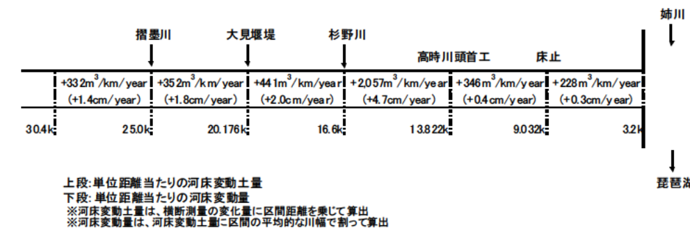
図 5.1.3 単位距離当たりの年平均河床変動土量
