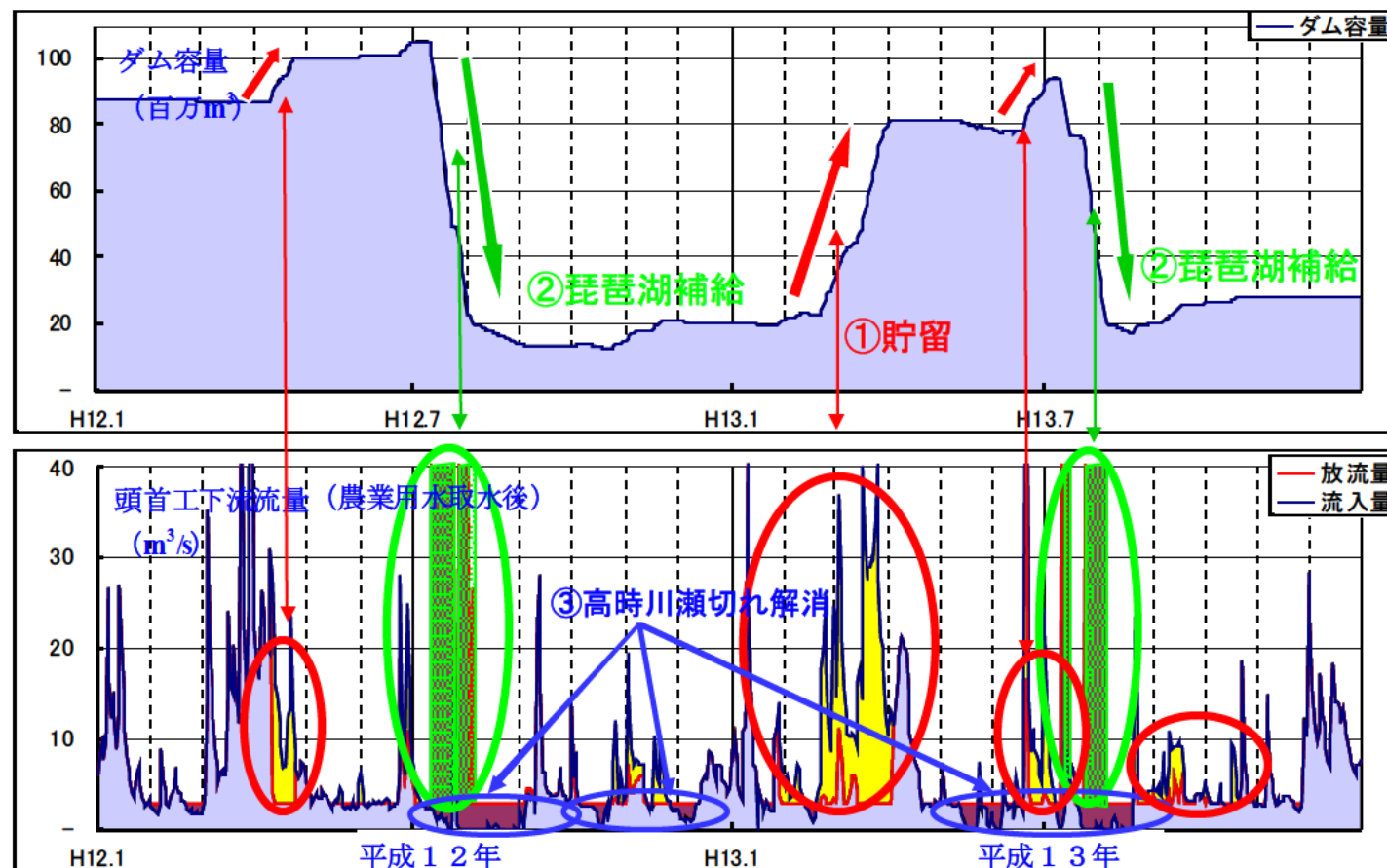
図 2.1.4 丹生ダムの容量と高時川頭首工下流流量 (平成 12 年～平成 13 年)
