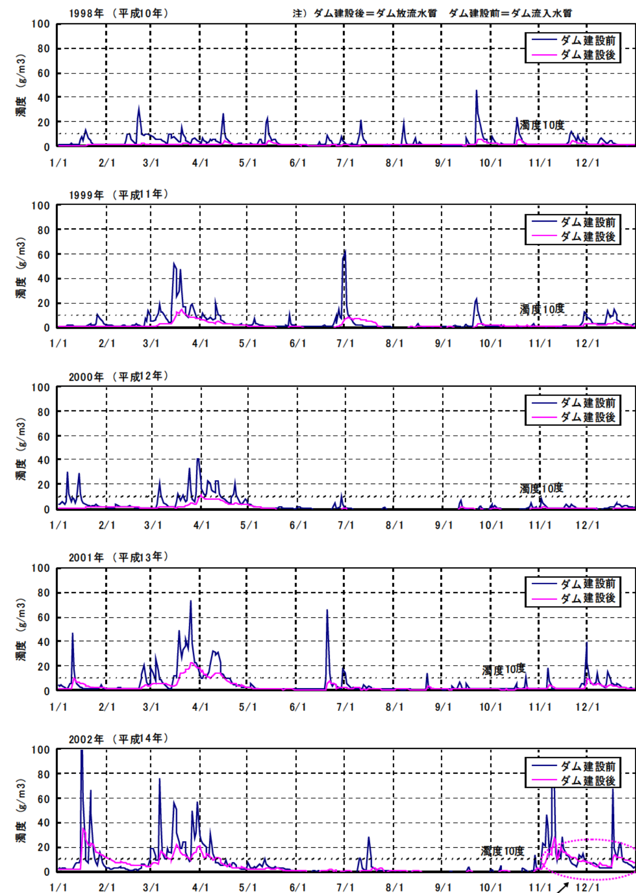
図 4.1.11 丹生ダム水質計算結果（濁度：1998～2002 年）
