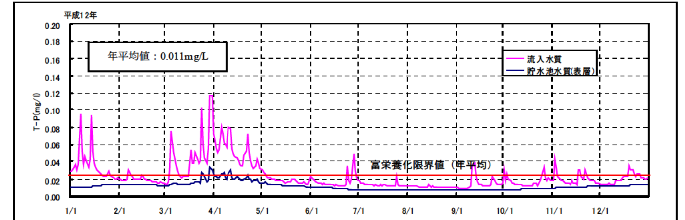
図 4.1.6 丹生ダム貯水池水質の予測結果の一例（2000 年）
