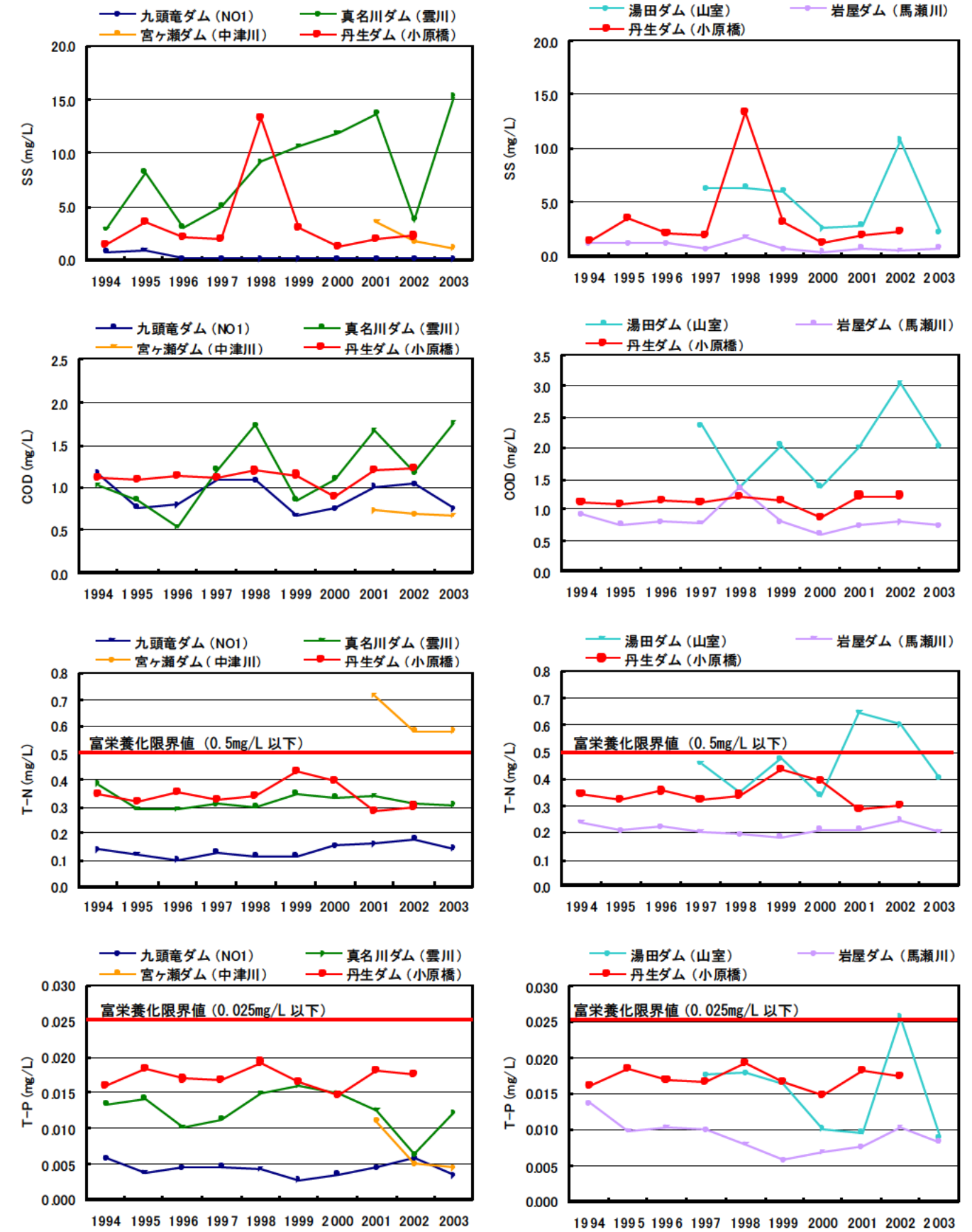
図 4.1.17 各ダム貯水池の流入水質レベルの比較（年平均値の動向）
