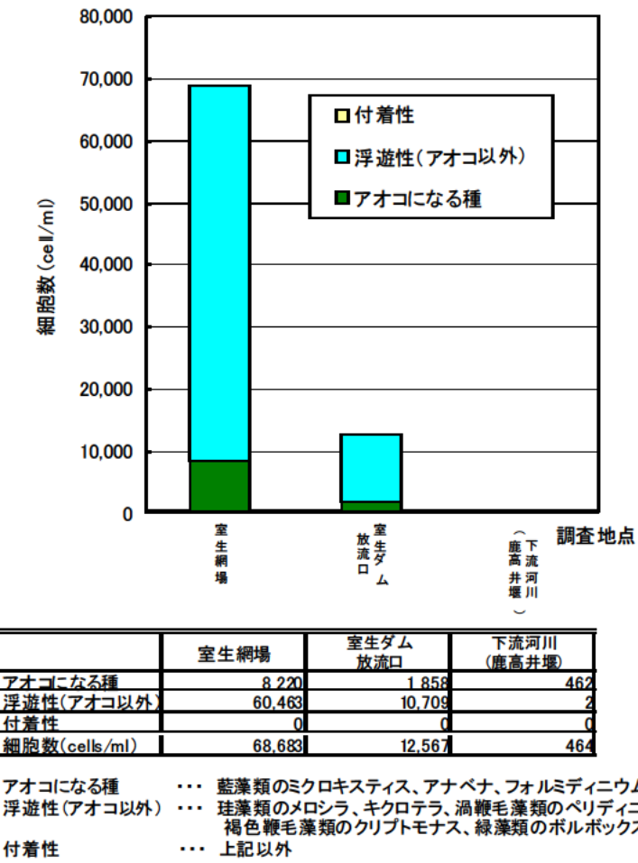
図 4.1.15 ダム貯水池表層と下流河川における植物プランクトン現存量の比較 (H14 年 9 月 24 日調査結果)
