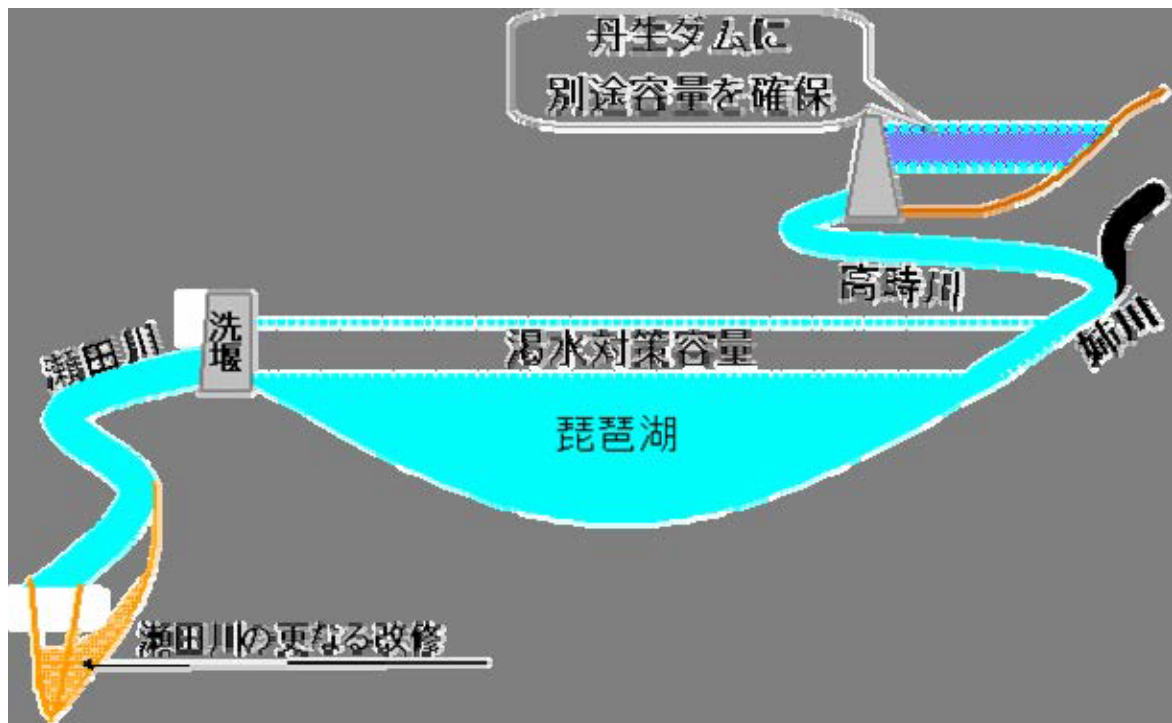
図 2 3 新たなダム方針における瀬田川改修、渇水対策容量及び丹生ダム容量のイメージ
