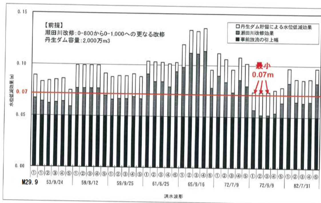
図2-2 水位上昇の抑制効果（低下量）
