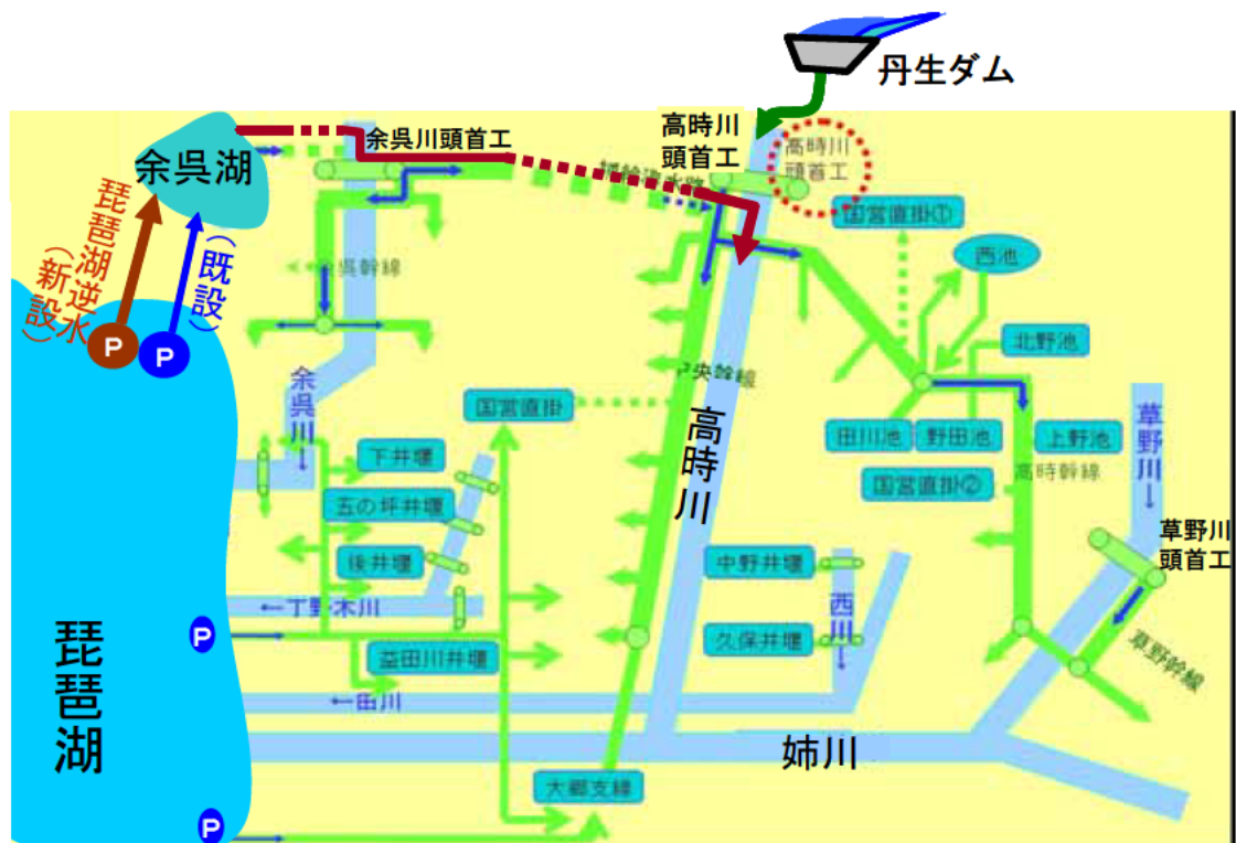
図 2 4 高時川の瀬切れ対策
