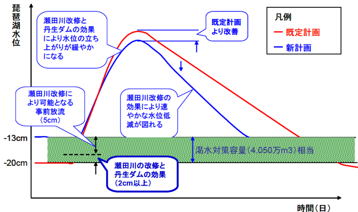
図 2 2 既定計画と新計画の琵琶湖水位の変化
