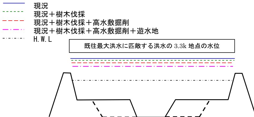
図 8 樹木伐採や高水敷掘削と遊水地の組合せの効果(既往最大洪水に匹敵する洪水)
