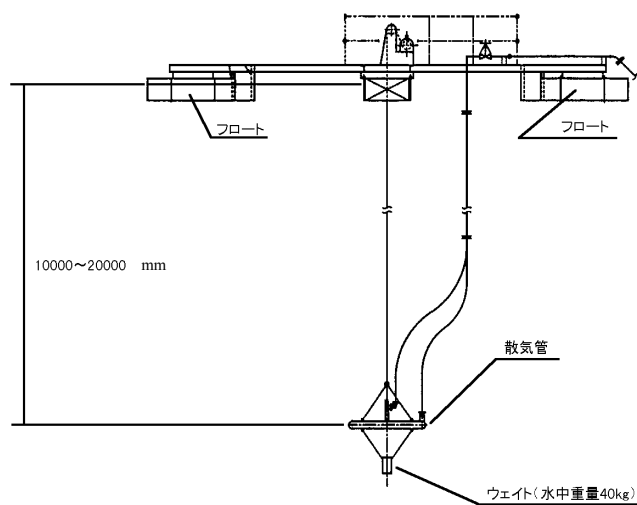
図 4.1.2 曝気装置概要図および曝気装置運転の様子（草木ダム）
