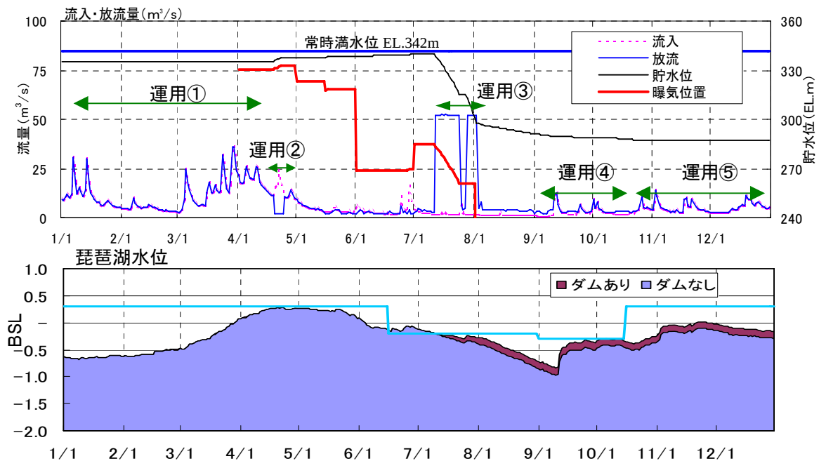
図 2.3.4 貯水位と曝気水深および琵琶湖水位の例（平成 12 年：2000 年）
