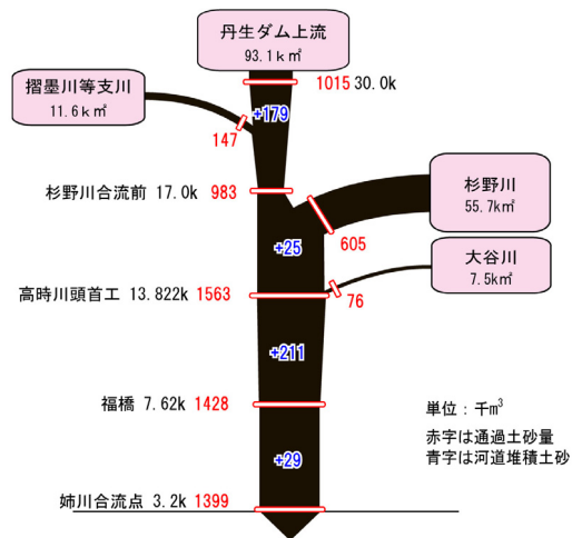
図 5.1.10 丹生ダムなし この差がダムによる土砂流出抑止効果 図 5.1.11 丹生ダムあり（洪水全量カット）
