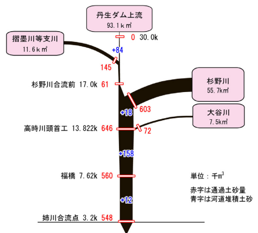
図 5.1.10 丹生ダムなし この差がダムによる土砂流出抑止効果 図 5.1.11 丹生ダムあり（洪水全量カット）
