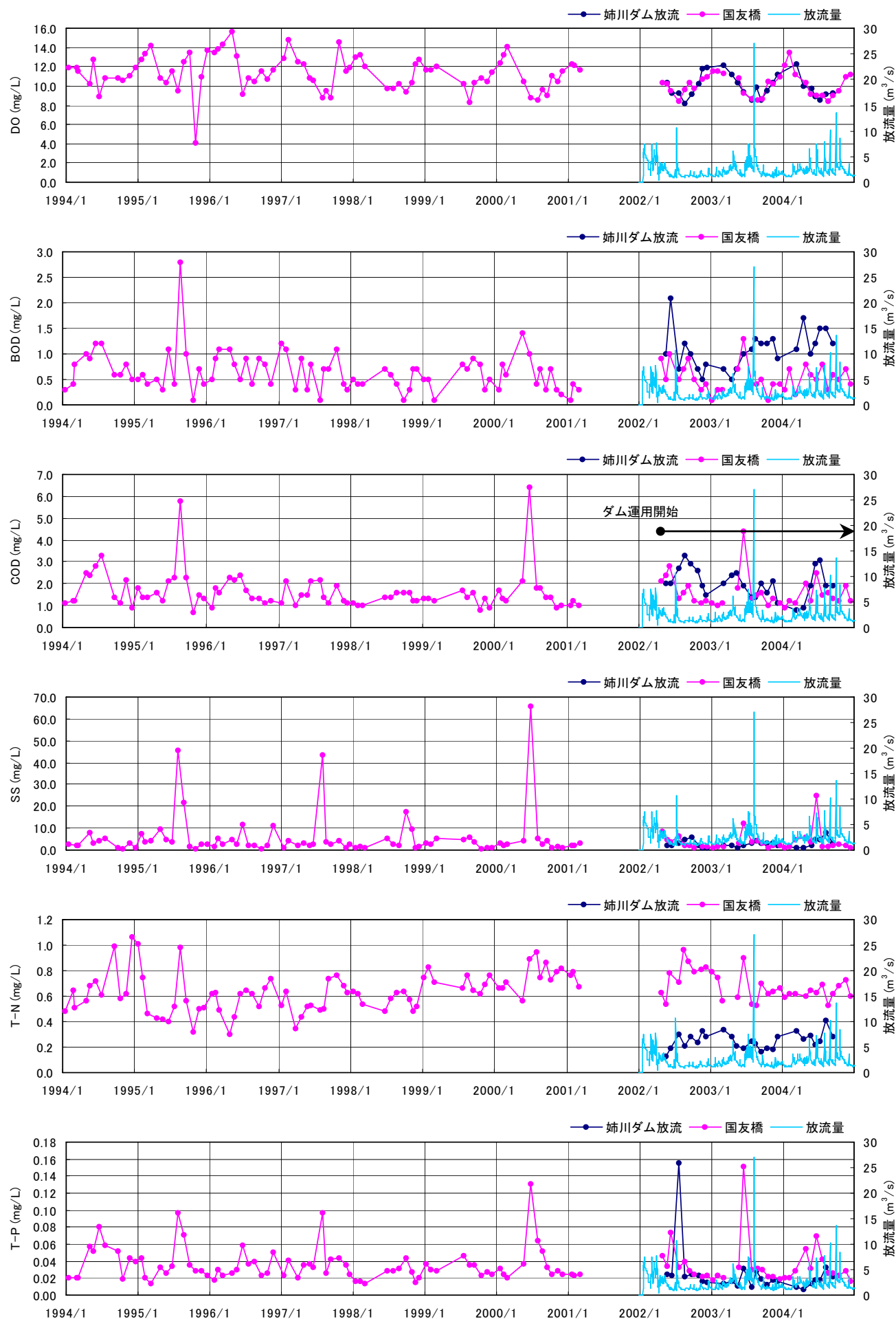
図 4.1.14 姉川ダム放流水質と姉川下流水質（国友橋）の関係
