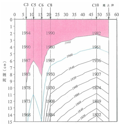
図 6.1.6 堆積年代算定結果
