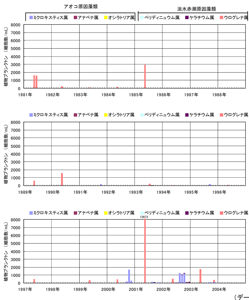
図 4.1.13 北湖安曇川沖中央地点におけるアオコおよび淡水赤潮の原因となる種の現存量の推移 (表層)
