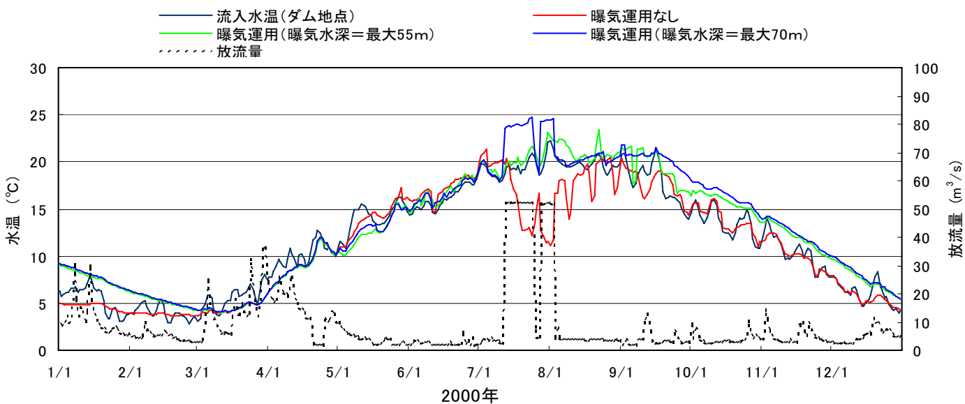
図 4.1.3 選択放流取水設備および曝気循環設備運用による水温の予測結果（2000 年）
