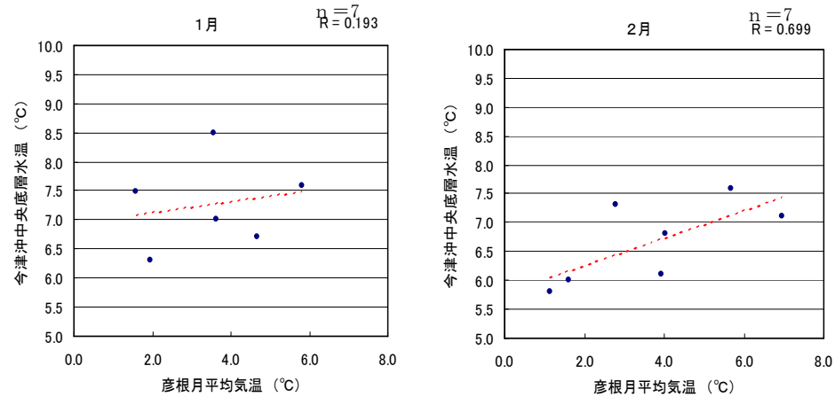
図 3.1.2 琵琶湖完全循環期（1～2 月）における月平均気温と各地点底層水温の関係（その 1）
