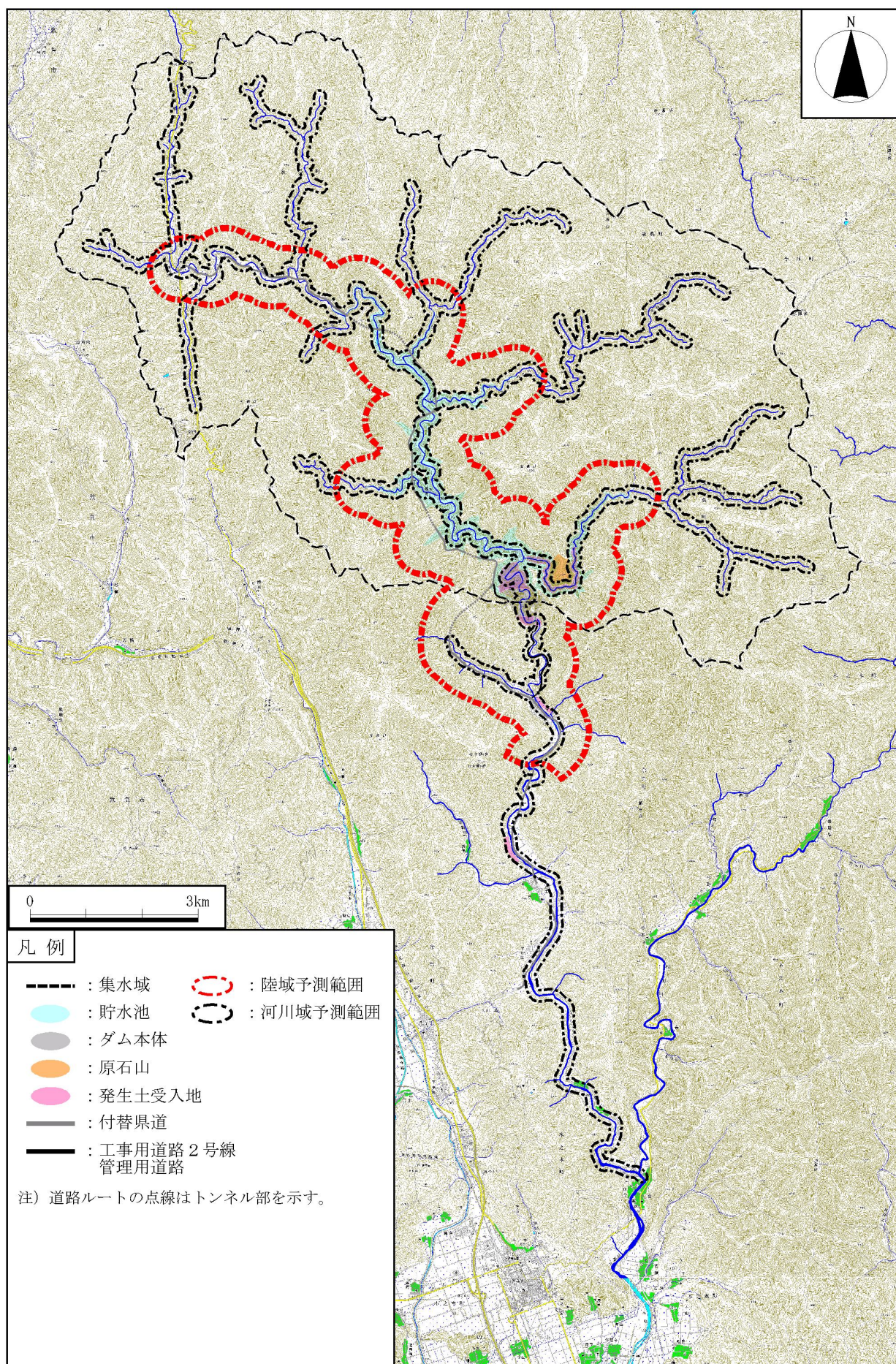
図－3 重要な種（動物）の影響予測範囲
