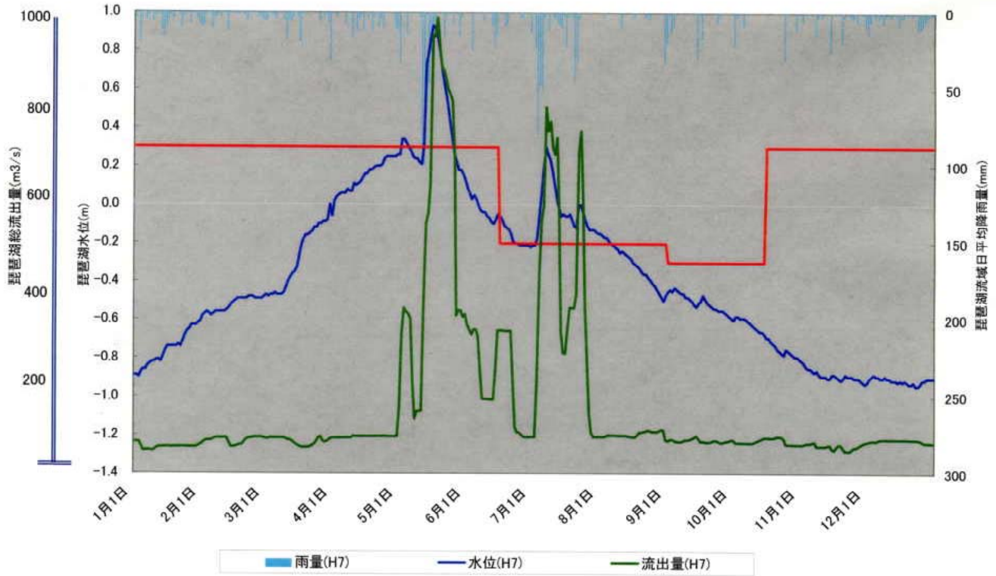
琵琶湖水位・降雨量・流出量〔平成7年〕
