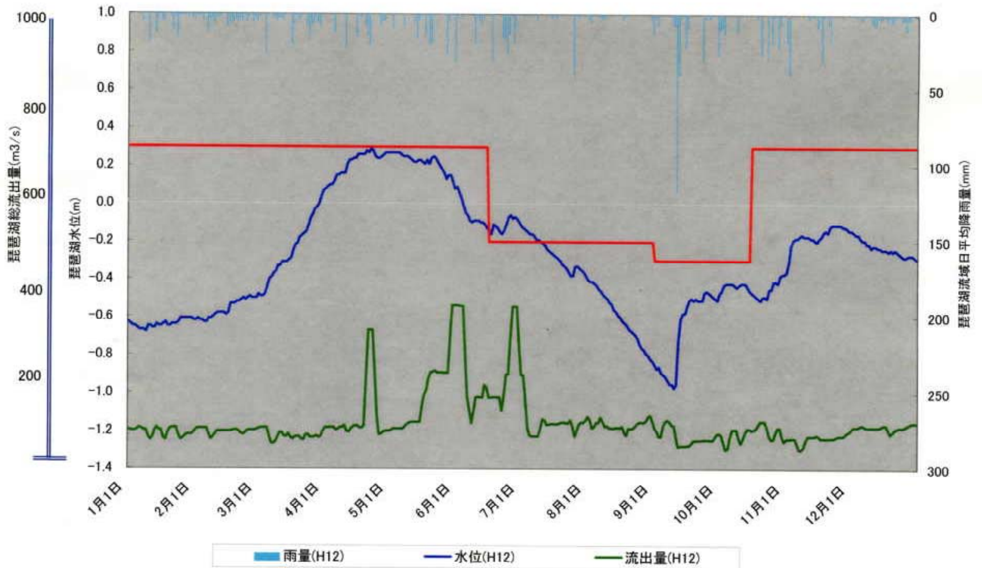
琵琶湖水位・降雨量・流出量〔平成12年〕
