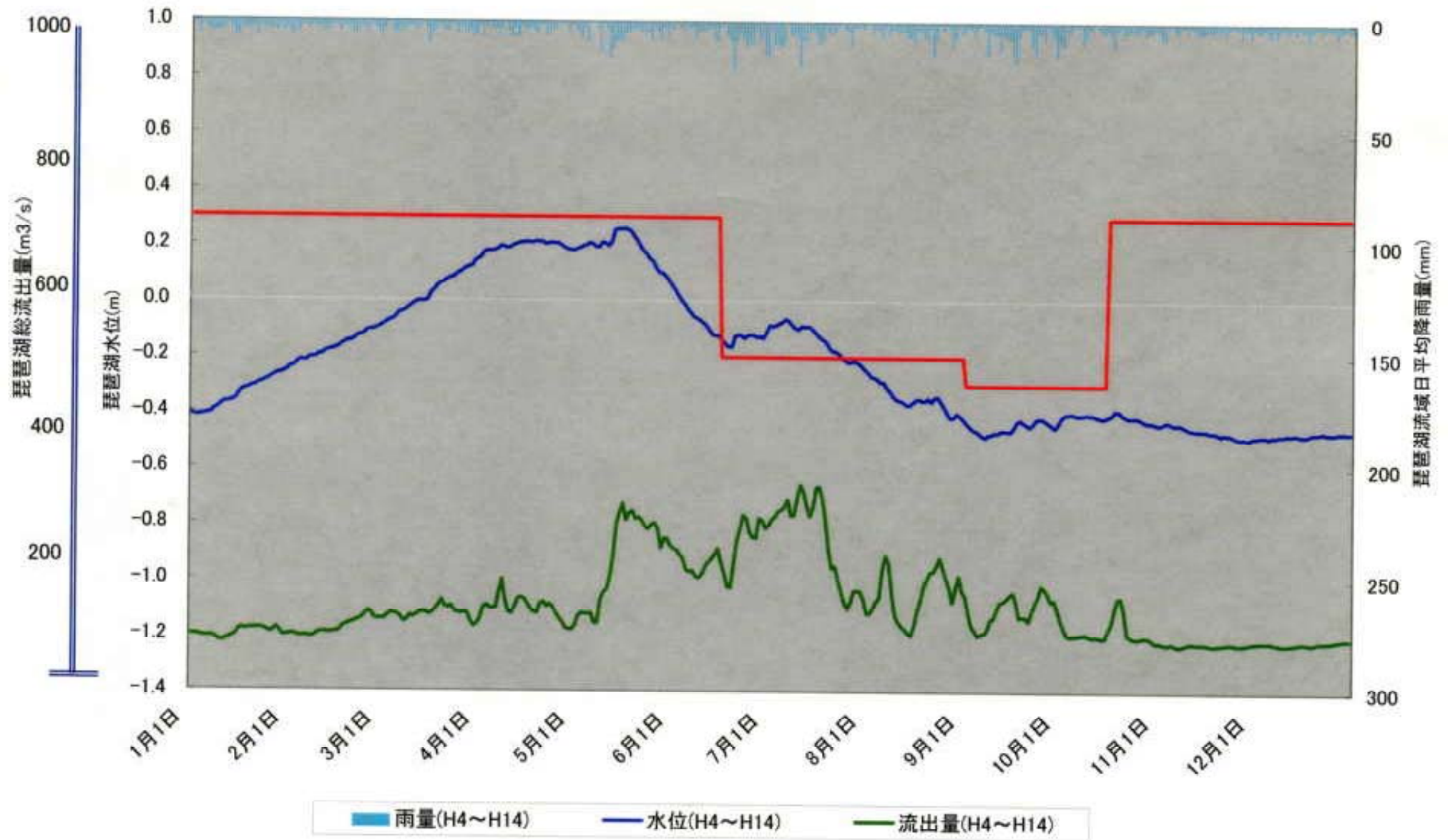
琵琶湖水位・降雨量・流出量〔平成4～14年平均〕
