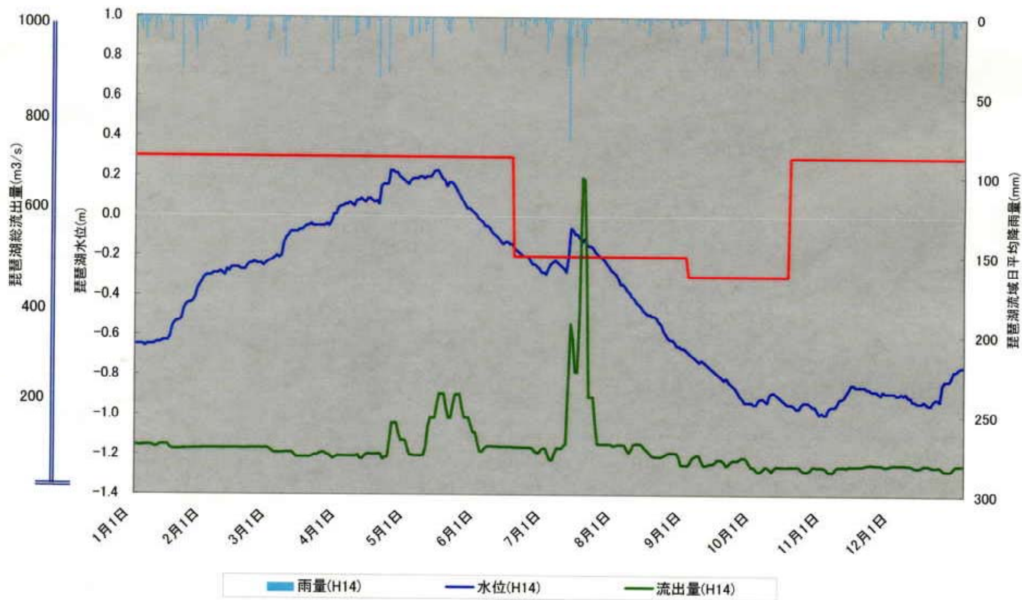
琵琶湖水位・降雨量・流出量〔平成14年〕
