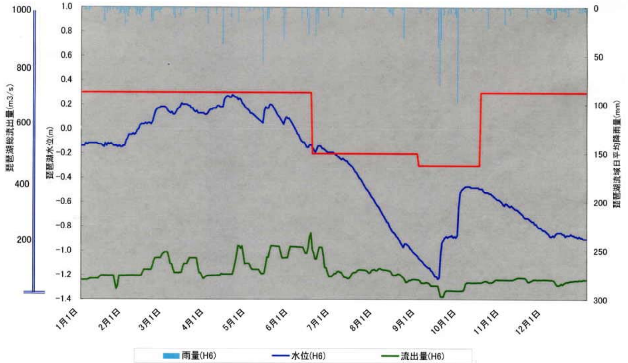
琵琶湖水位・降雨量・流出量〔平成6年〕
