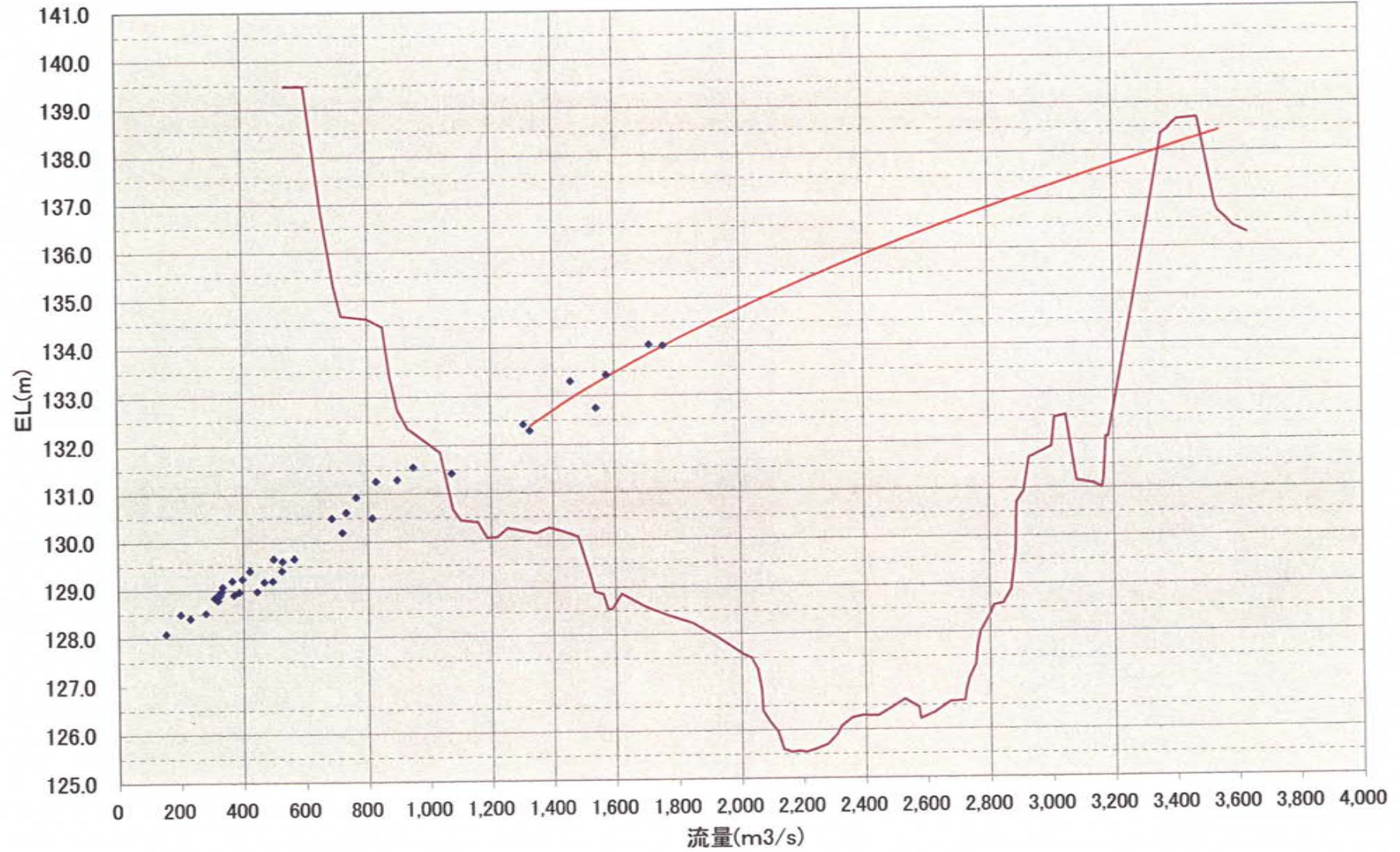
岩倉(57.4km)地点水位流量曲線図
