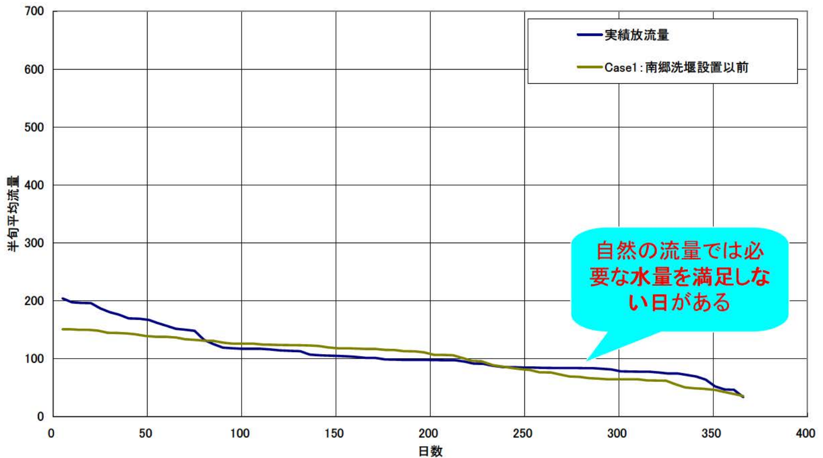
琵琶湖放流量流況曲線(渇水年H6年)
