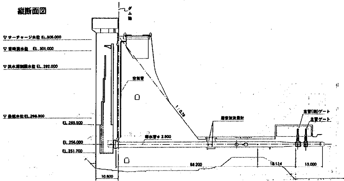
図-1.3.5 低水放流設備
