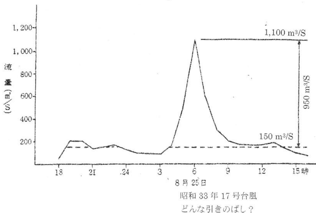
No. 15 図 洪水調節図(川上ダム地点)
