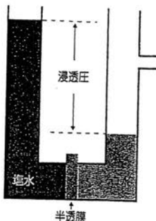
(2) 浸透平衡
