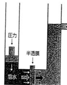
(3) 逆浸透現象
