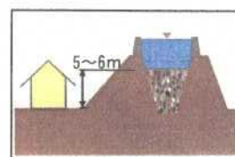
旧草津川の 堤防断面
