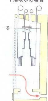
下層取水の場合
