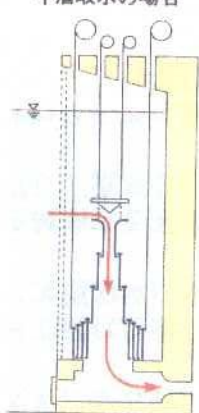
中層取水の場合
