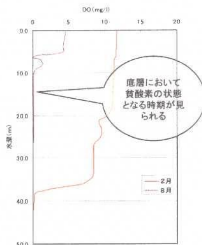
平成14年室生ダムDO分布
