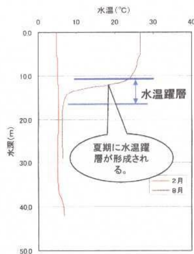
平成14年室生ダム水温分布
