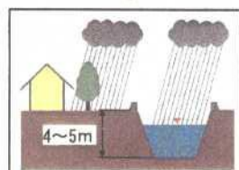
草津川放水路の 堤防断面
