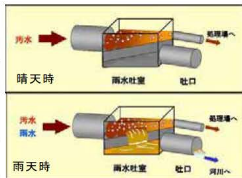
図 2 1 2 合流式下水道の晴天時、雨天時の水の流れ
