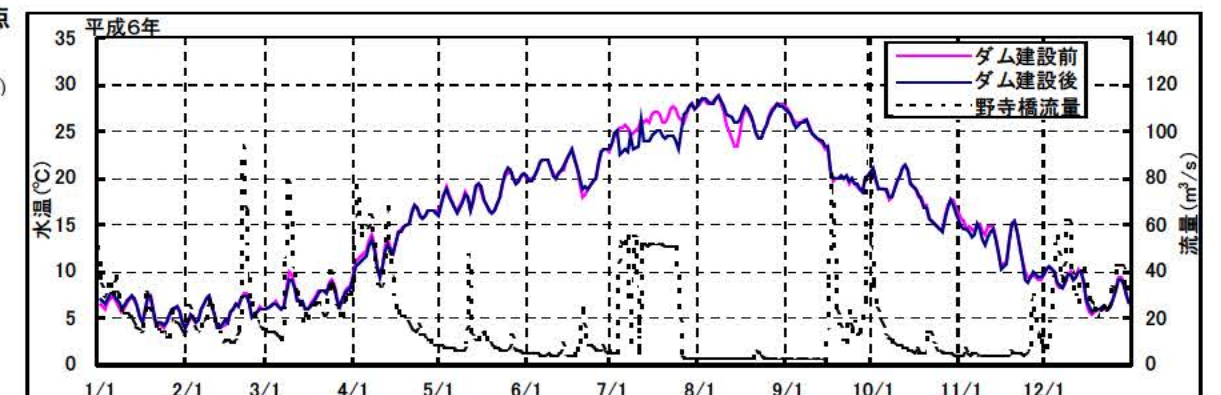
図 4.1.8 ダム下流河川水温予測結果（1994 年：選択取水・曝気あり、環境放流実施）
