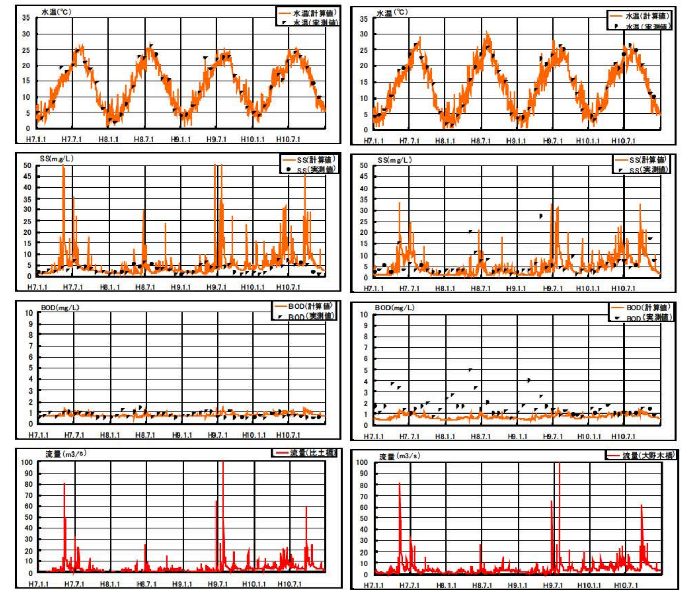
図 2.1.2(1) 下流河川モデルの検証（平成7年～10年）
