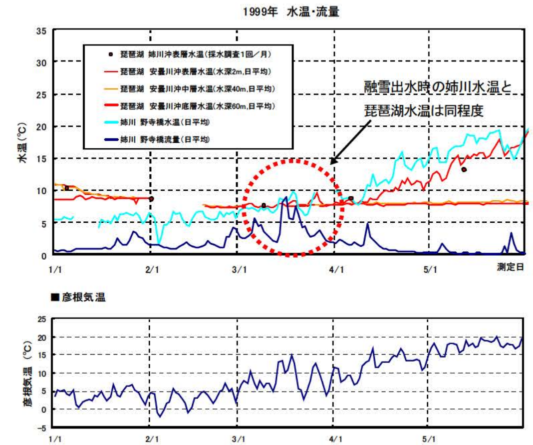
図 3.1.7 姉川水温と琵琶湖水温の関係（1999 年）
