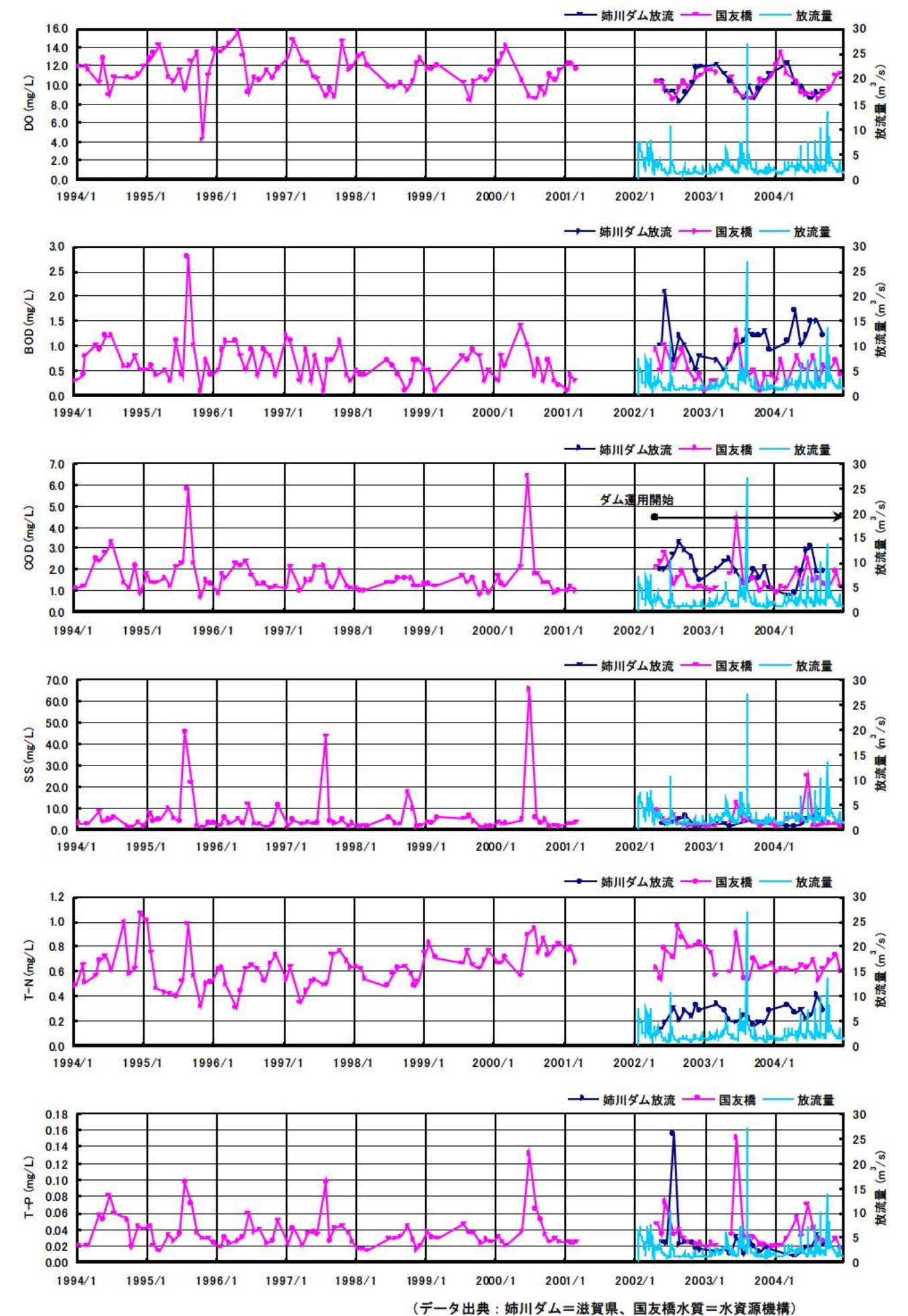
図 4.1.14 姉川ダム放流水質と姉川下流水質（国友橋）の関係
