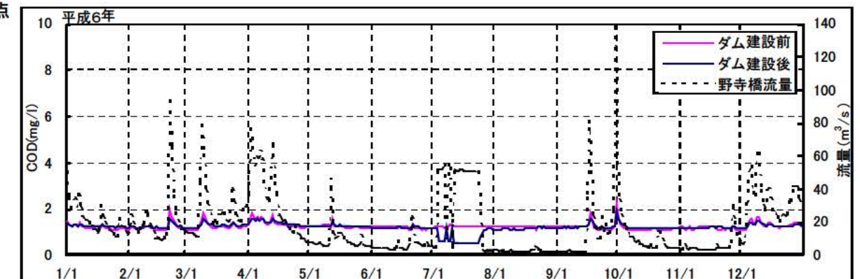
図 4.1.10 ダム下流河川 COD 予測結果 (1994 年: 選択取水・曝気あり、環境放流実施)
