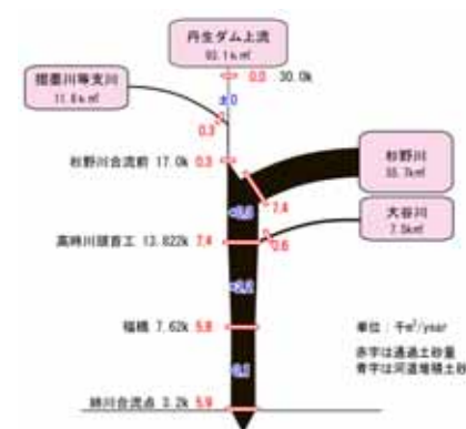
【参考】丹生ダムが洪水調節をしなかった場合（全流砂）
