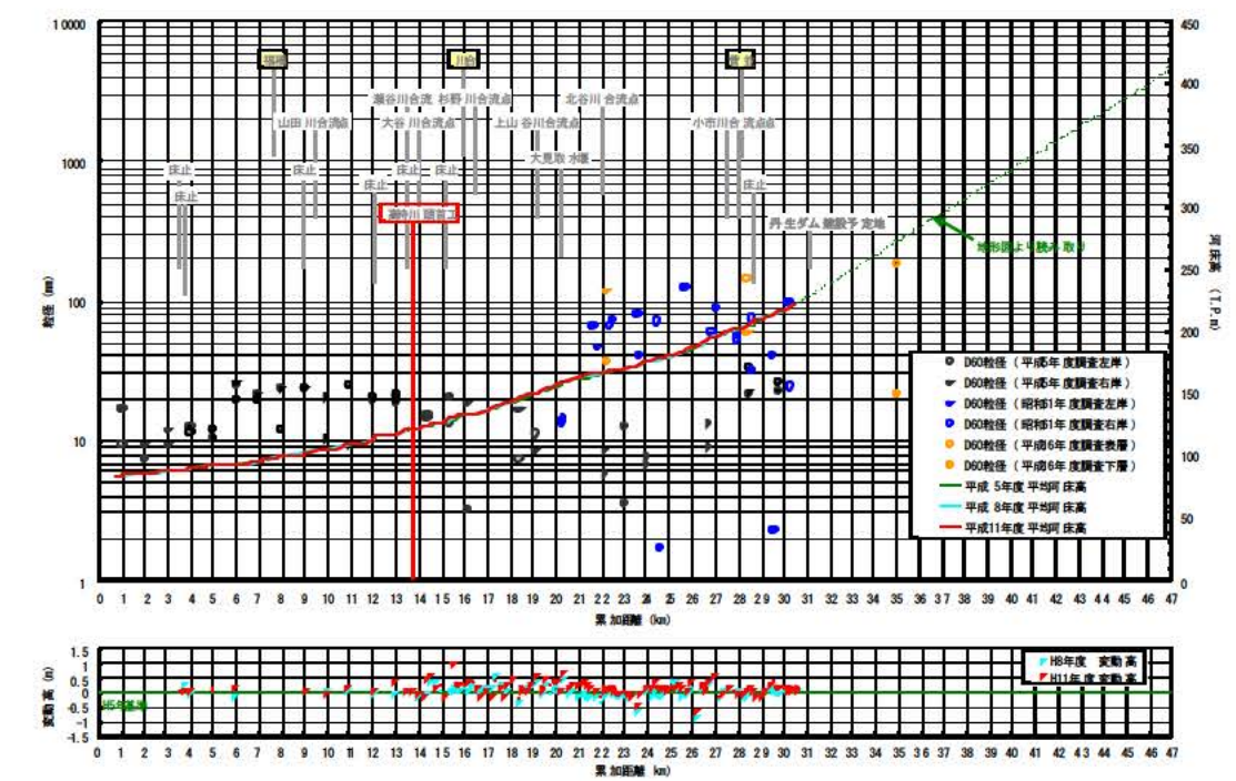
図 5.1.2 平均河床高と代表粒径の縦断図
