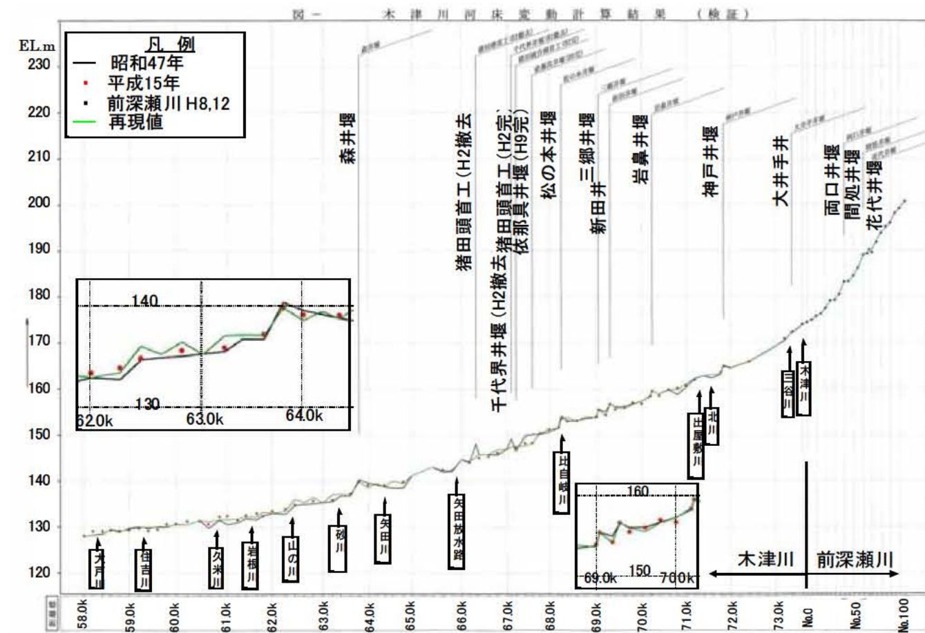
図 1.2.1 1次元河床変動解析モデルの検証（下流河川）
