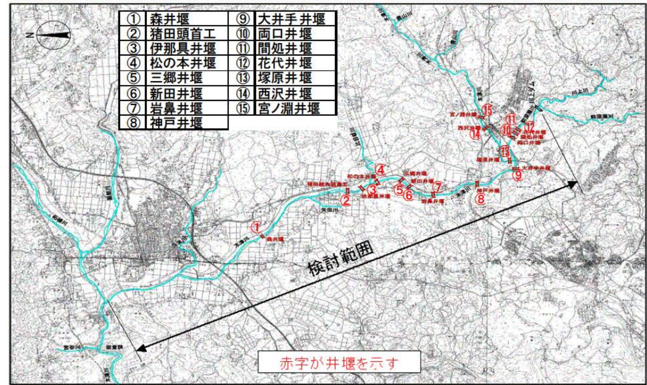
図 1.1.1 河川構造物分布位置図
