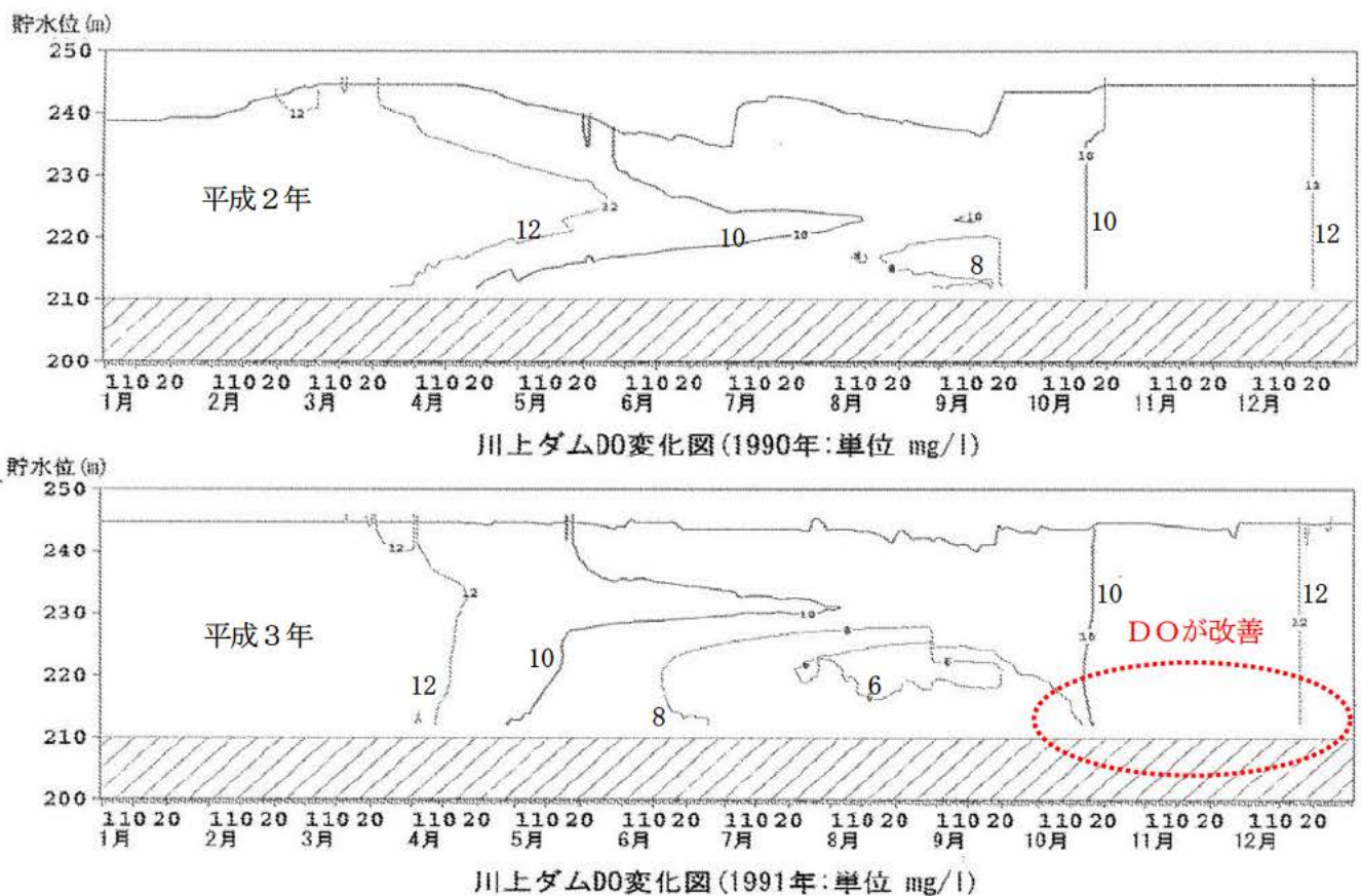
図 3.1.2 DOの鉛直分布時系列図(保全対策あり)
