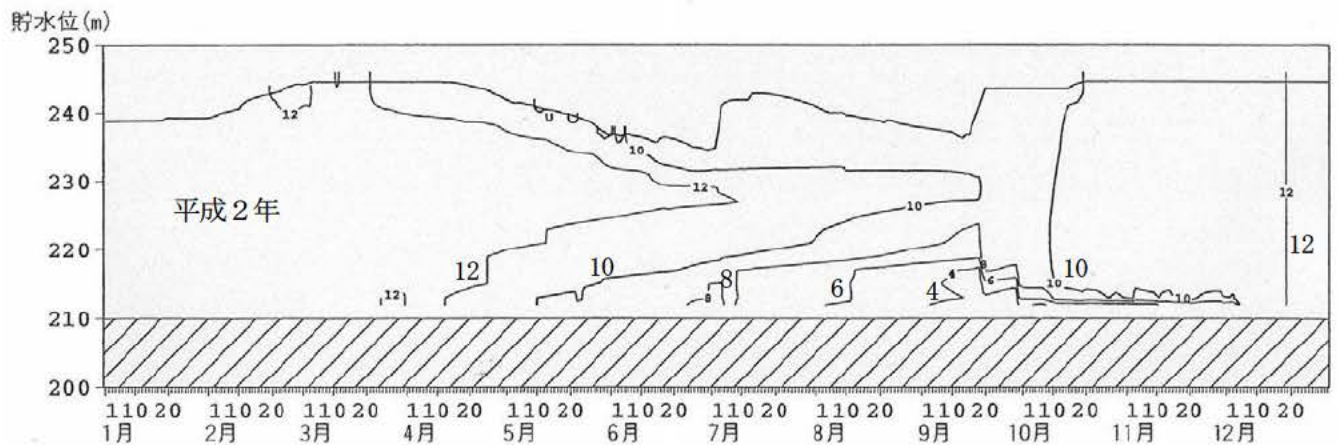
川上ダムDO変化図(1990年:単位 mg/l)
