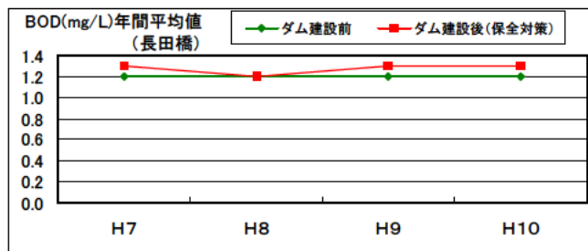
図 3. 1. 3 下流河川の水質・水温の経年変化 (保全対策あり)
