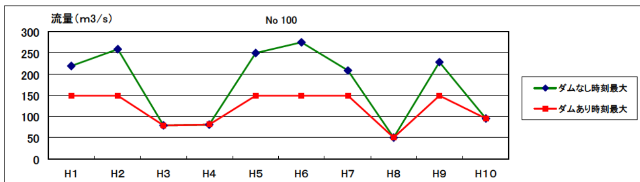
図 1. 1. 1 時刻最大流量の経年変化
