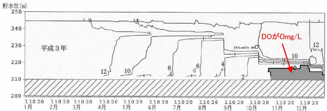
川上ダムDO変化図(1991年:単位 mg/l)
