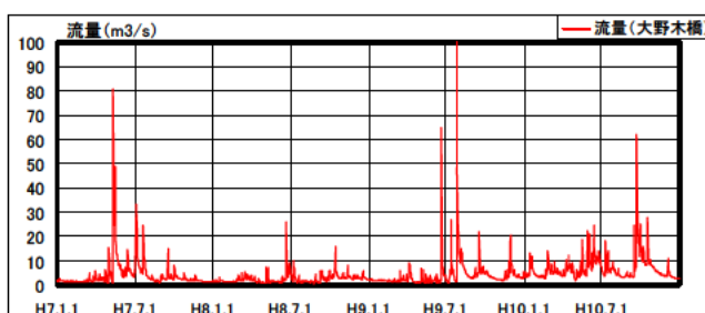
図 2.1.2(1) 下流河川モデルの検証 (平成7年～10年)
