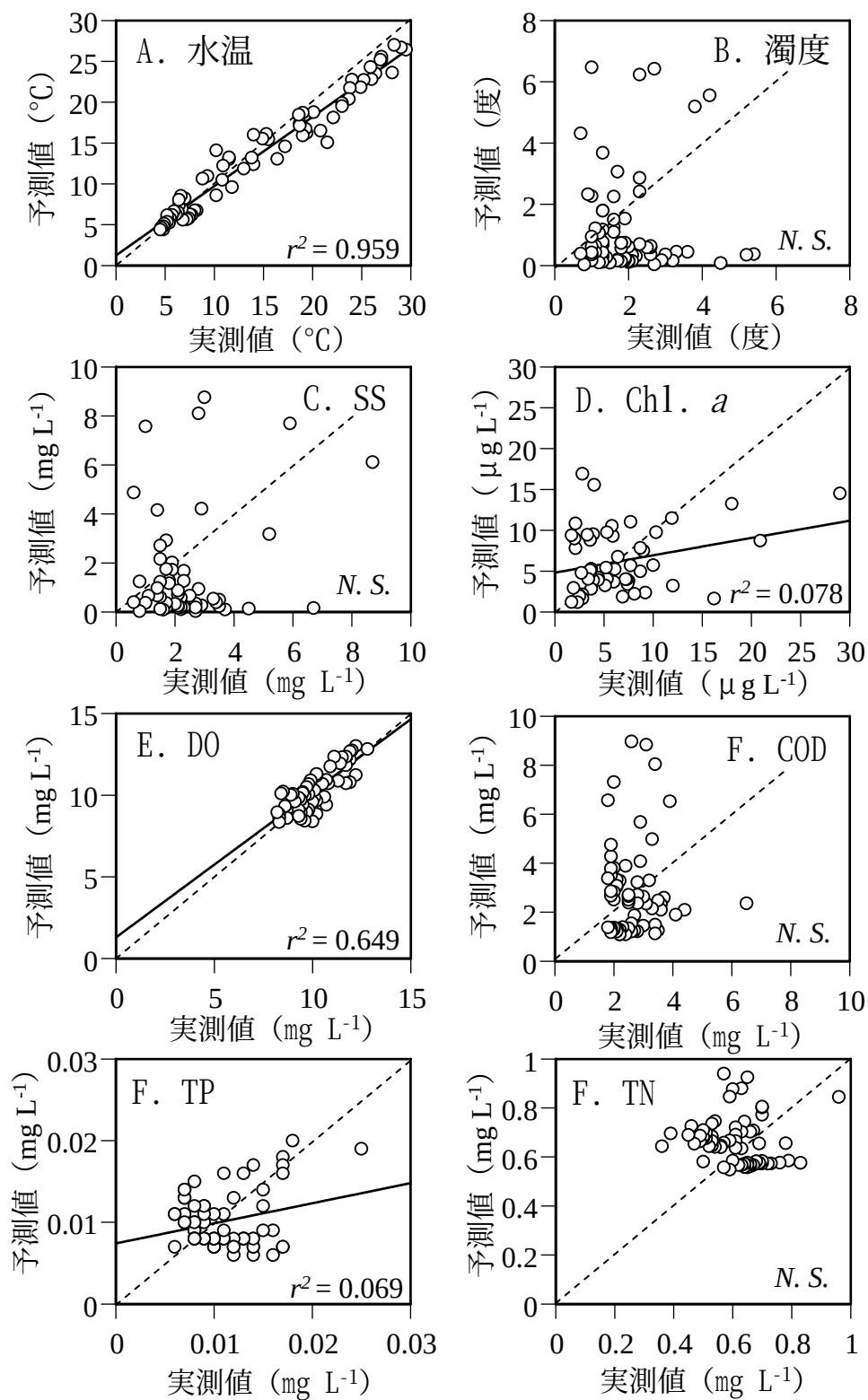
図1. 鉛直次元モデルによる比奈知ダムの水質予測値と実測値の関係 (図中の破線は y = x を、実線は回帰直線を示す)。
