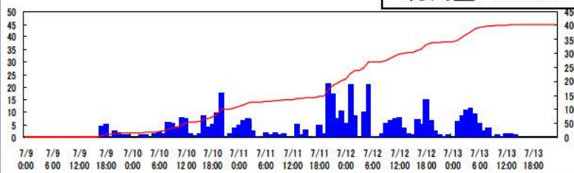
昭和47年7月洪水(丹生ダム流域)
