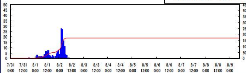
昭和57年7月洪水(丹生ダム流域)
