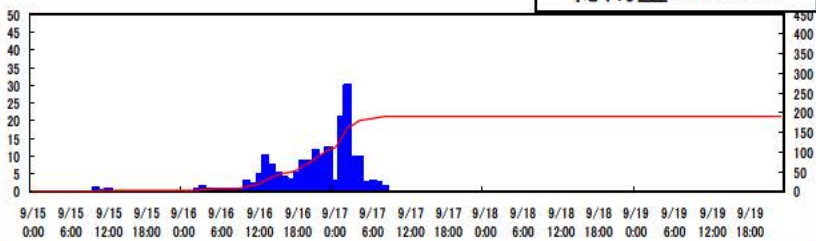
昭和47年9月洪水(丹生ダム流域)
