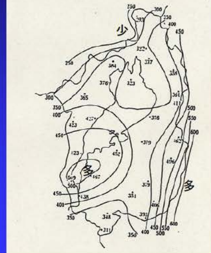
降水量分布図 昭和36年 6月24～29日
