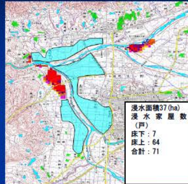
河床掘削・上野遊水地・川上ダム完成
