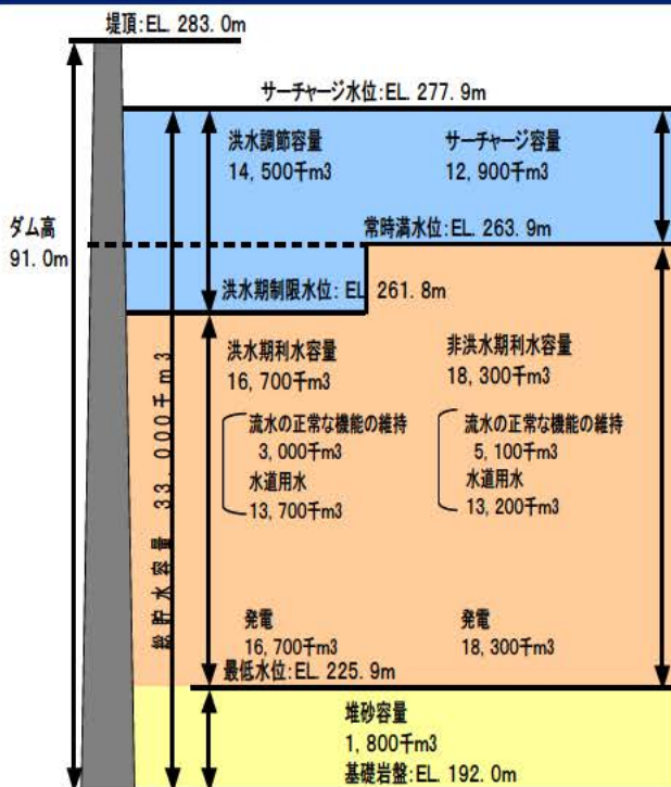
現計画 貯水池容量配分図
