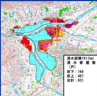
河床掘削・上野遊水地
