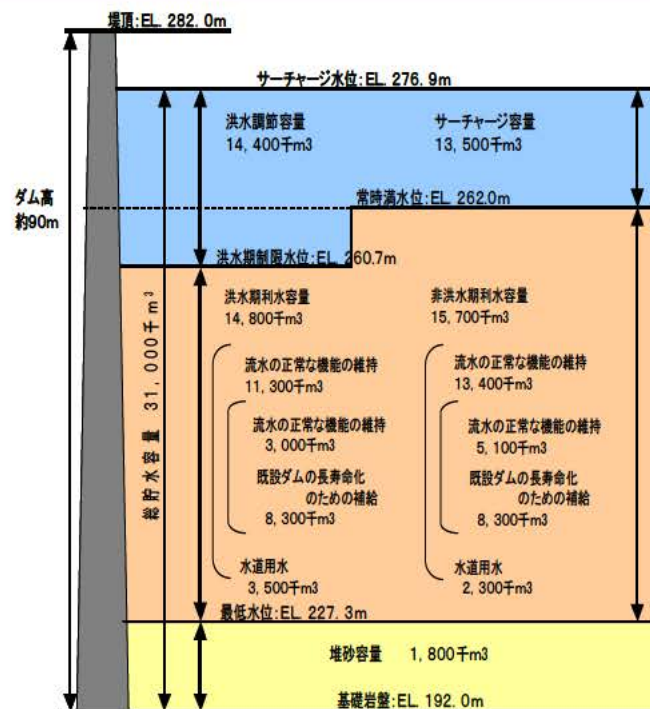
新計画 貯水池容量配分図
