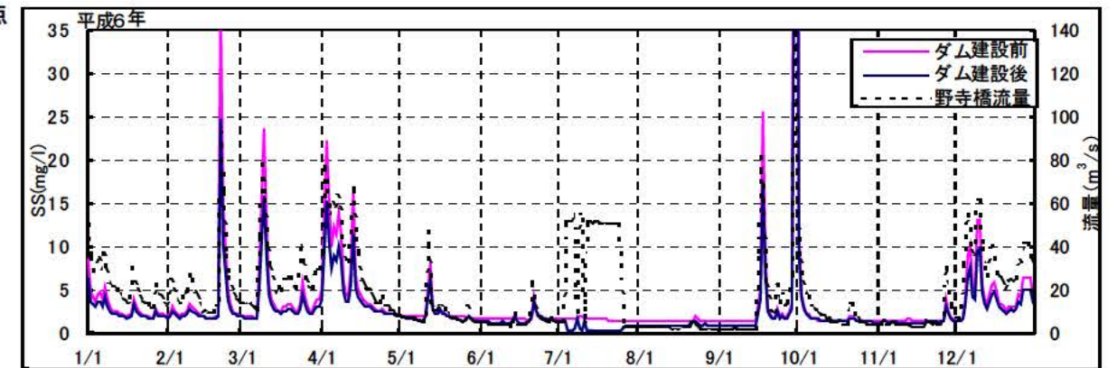
図 4.1.9 ダム下流河川SS予測結果（1994年：選択取水・曝気あり、環境放流実施）
