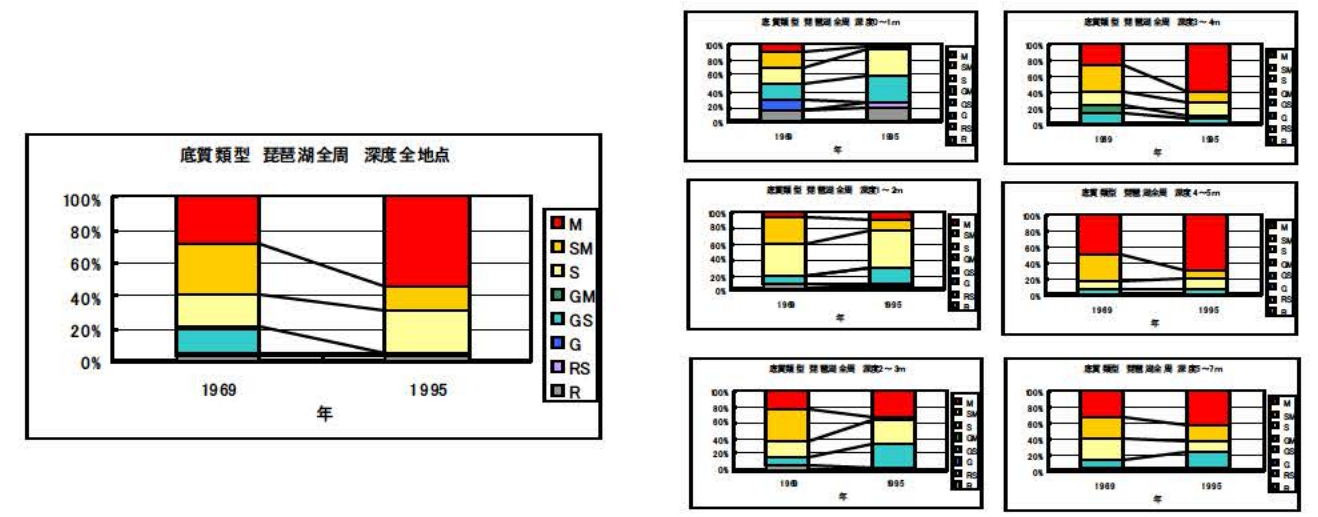
図 6.1.2 琵琶湖全周（底質面積の変化）
