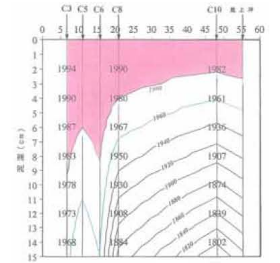
図 6.1.6 堆積年代算定結果
