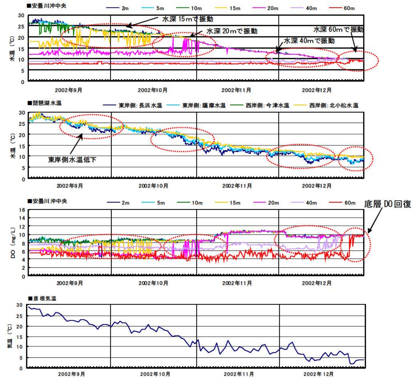
【出典】安曇川沖自動観測データ：水資源機構、琵琶湖水温：滋賀県、彦根気温：気象庁
