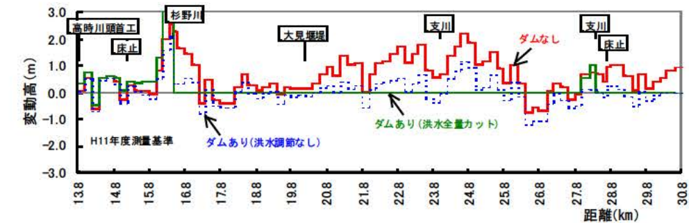
図 5.1.5 山地部における河床変動高予測結果（30 年間の予測計算）
