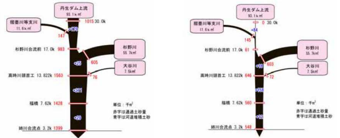
この差がダムによる土砂流出抑制効果 図 5.1.10 丹生ダムなし 図 5.1.11 丹生ダムあり（洪水全量カット）
