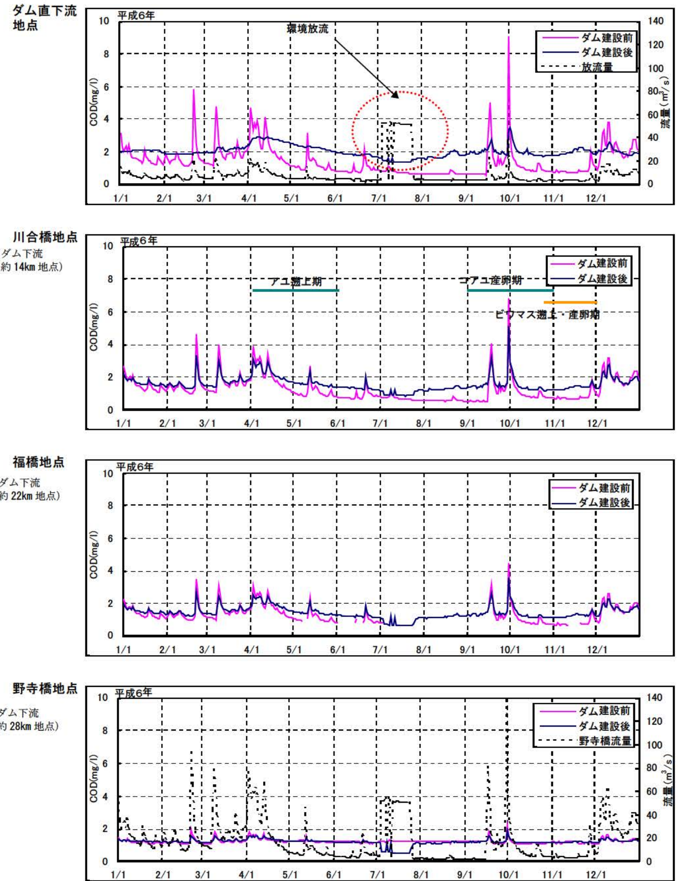
図 4.1.10 ダム下流河川COD予測結果 (1994年: 選択取水・曝気あり、環境放流実施)
