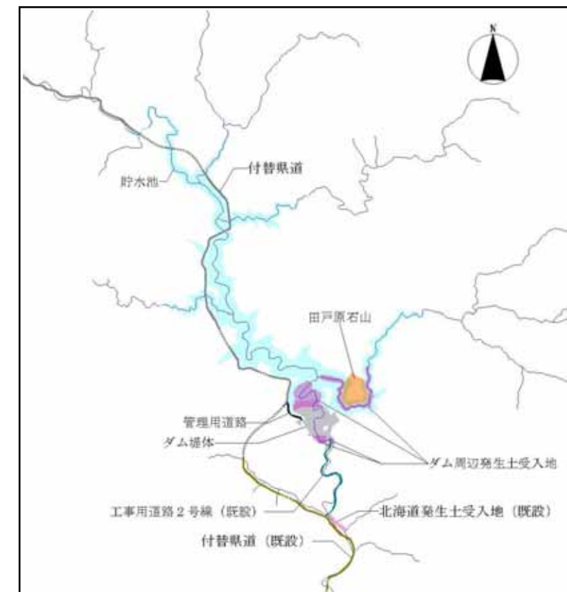
図 - 2 丹生ダム事業レイアウト
