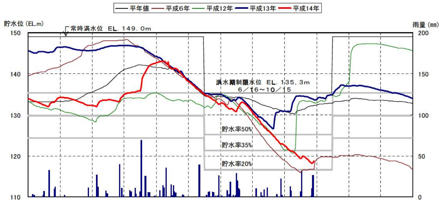
一庫ダム貯水位曲線
