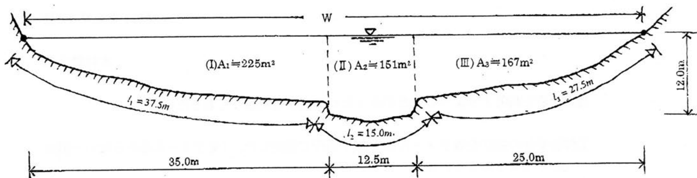
1) - d 流体横断面図 (しあん橋下流 50m 地点)
