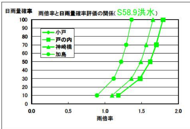
図-3 各洪水の雨倍率と日雨量確率評価の関係
