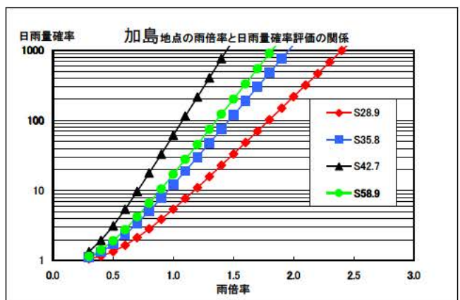
図-1 各地点の雨倍率と日雨量確率評価の関係 (対数グラフ)
