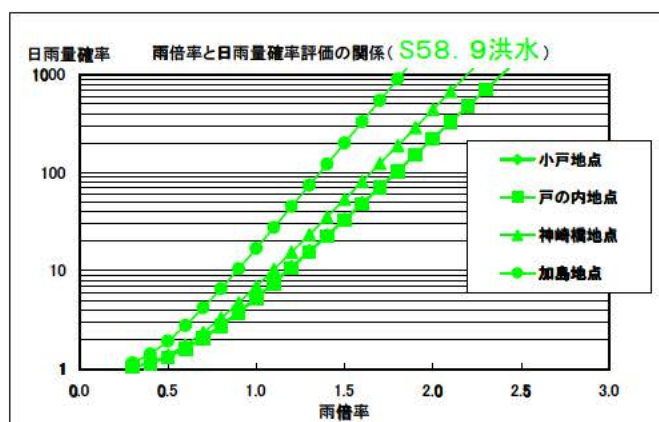
図-2 各洪水の降雨倍率と確率年の関係 (対数グラフ)
