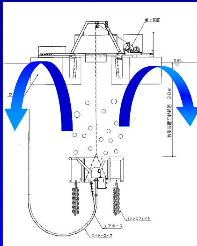
浅層曝気設備構造図
