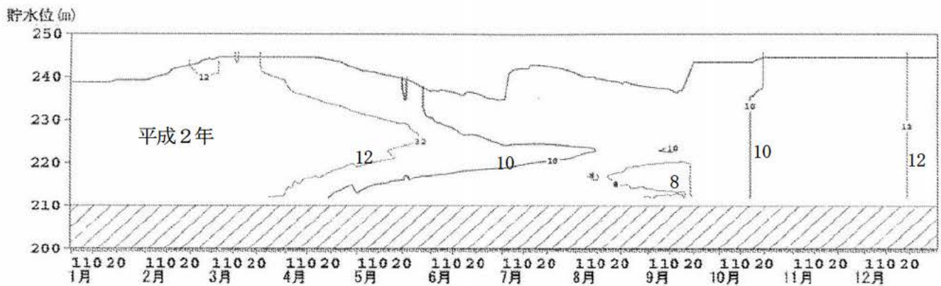
川上ダムDO変化図(1990年:単位 mg/l)
