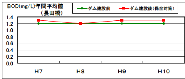
図 3. 1. 3 下流河川の水温・水質の経年変化(保全対策あり)
