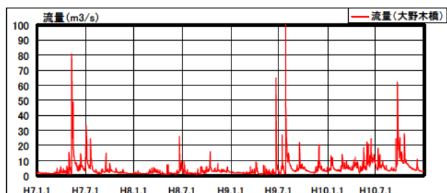
図 2. 1. 2(1) 下流河川モデルの検証 (平成 7 年～10 年)
