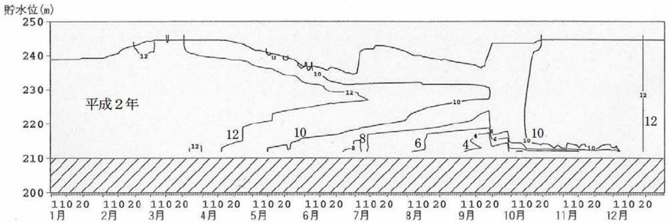
川上ダムDO変化図(1990年:単位 mg/l)
