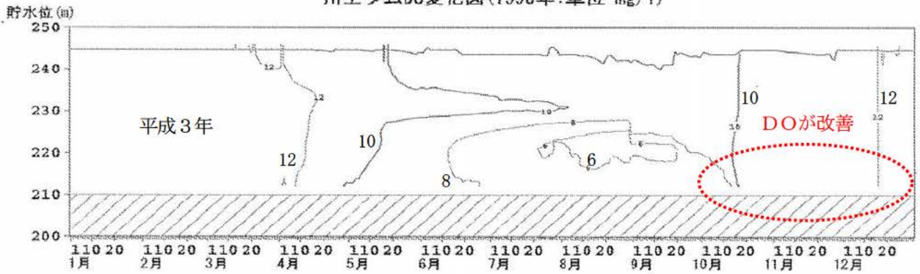
川上ダムDO変化図(1991年:単位 mg/l)
