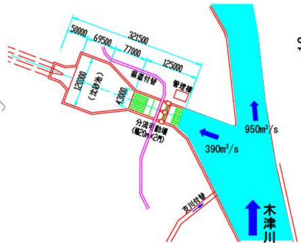
【呑口平面図】
