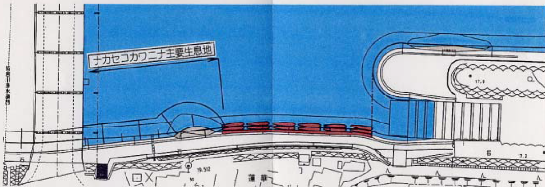
橘島低水護岸基礎位置までの配置案
