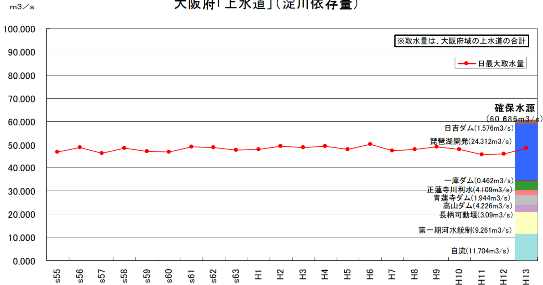
大阪府「上水道」(淀川依存量)
