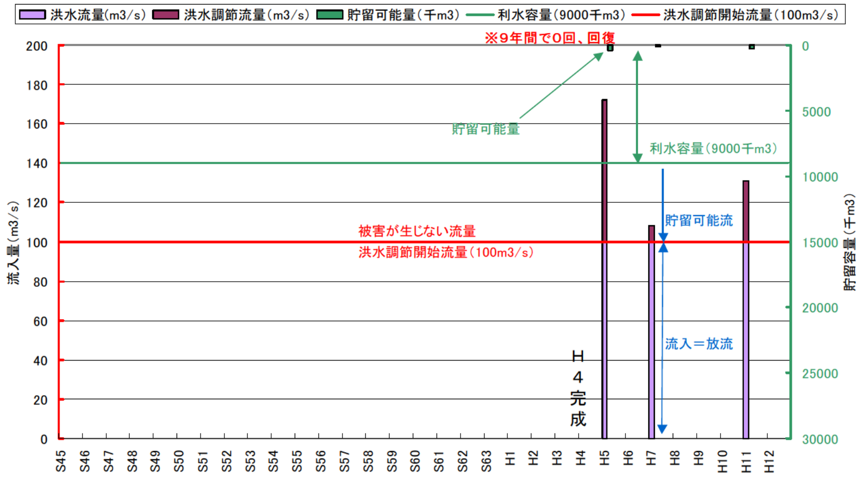
布目ダムの流量調整の可能性 (H4完成)
