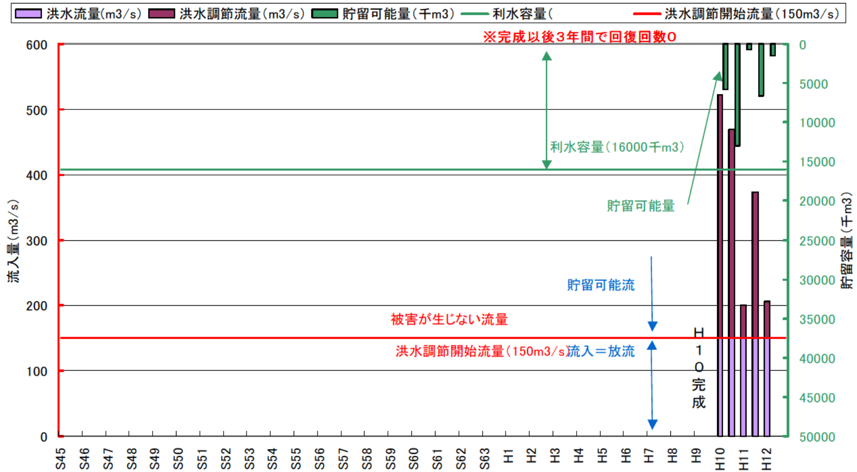
日吉ダムの流量調整の可能性 (H10年完成)
