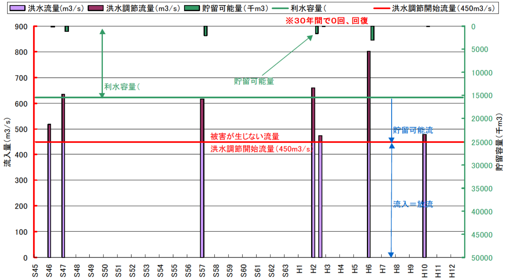
青蓮寺ダムの流量調整の可能性 (S45完成)
