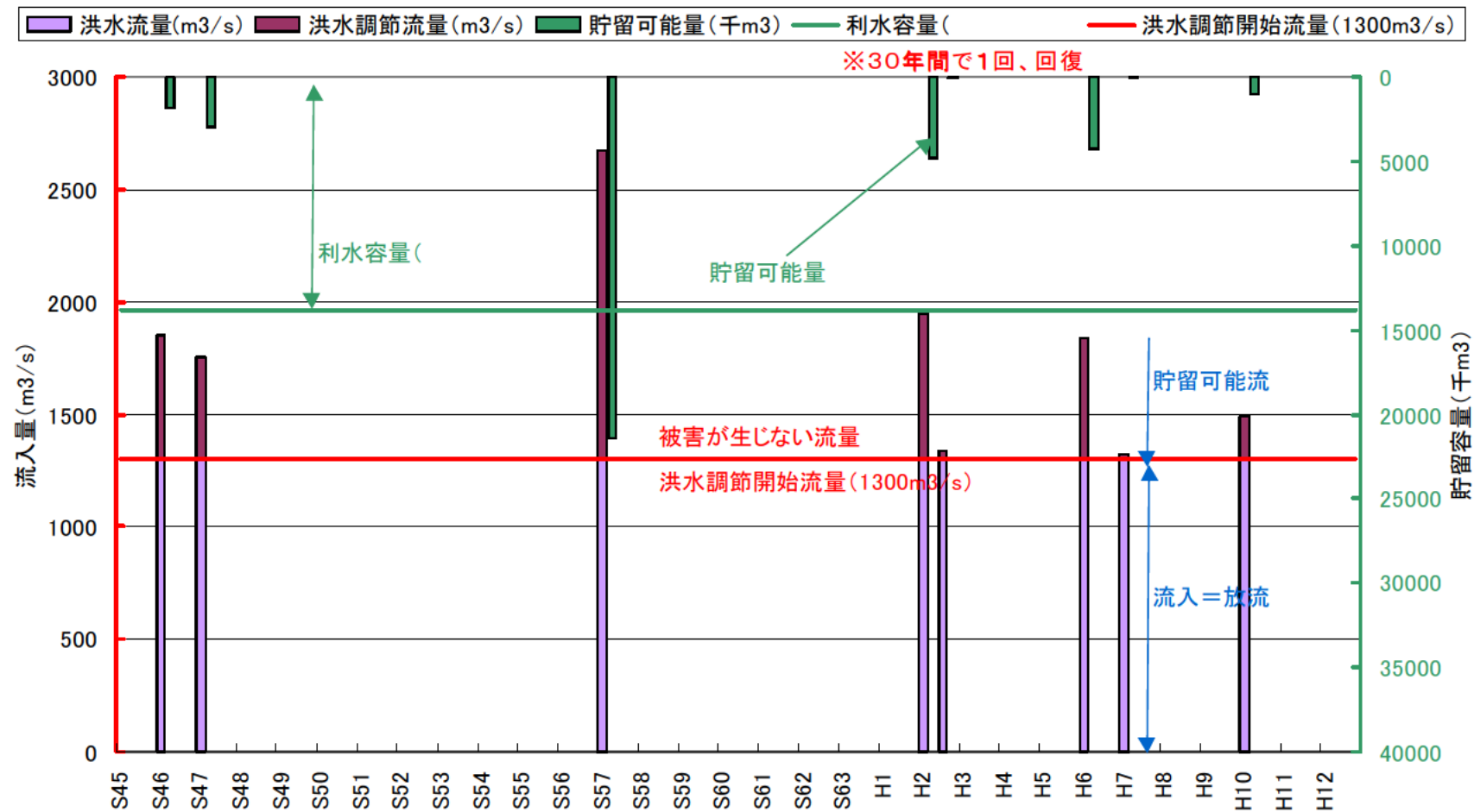
高山ダムの流量調整の可能性
