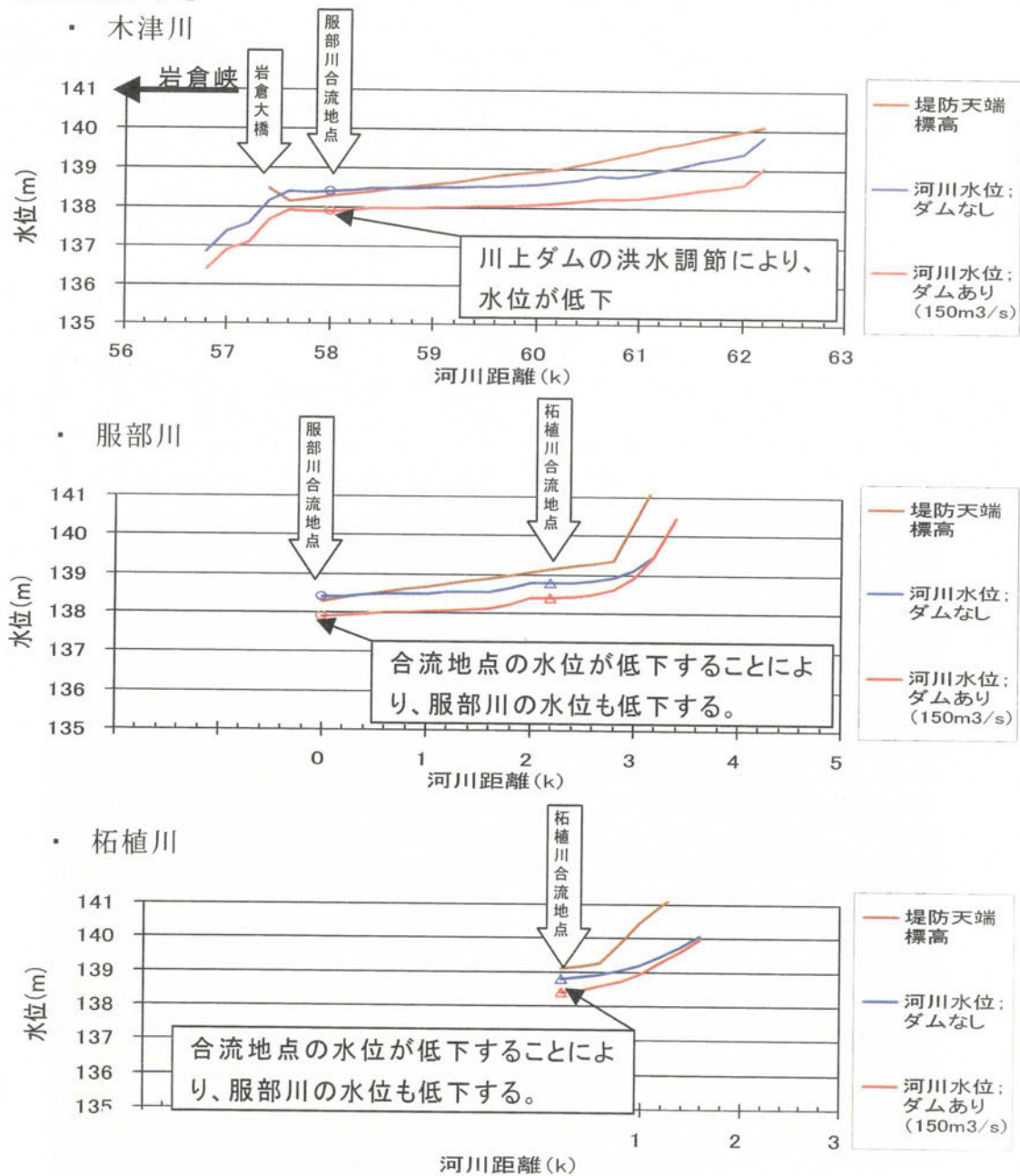
【水位縦断図】
