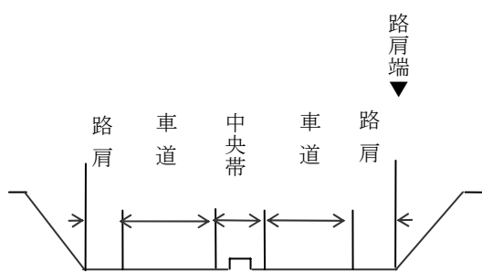
3) 切土構造
