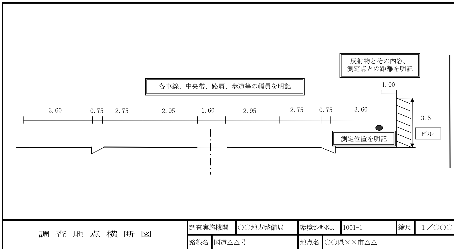
図 7.4.2 調査地点横断面図様式（記載例）
