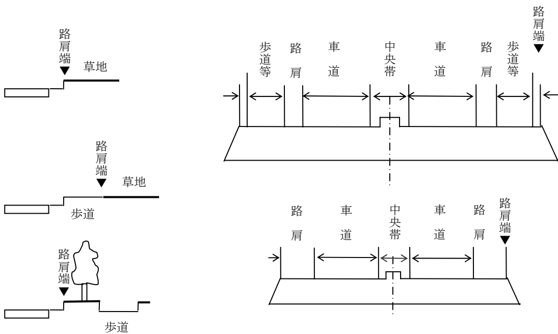
1) 平面構造
