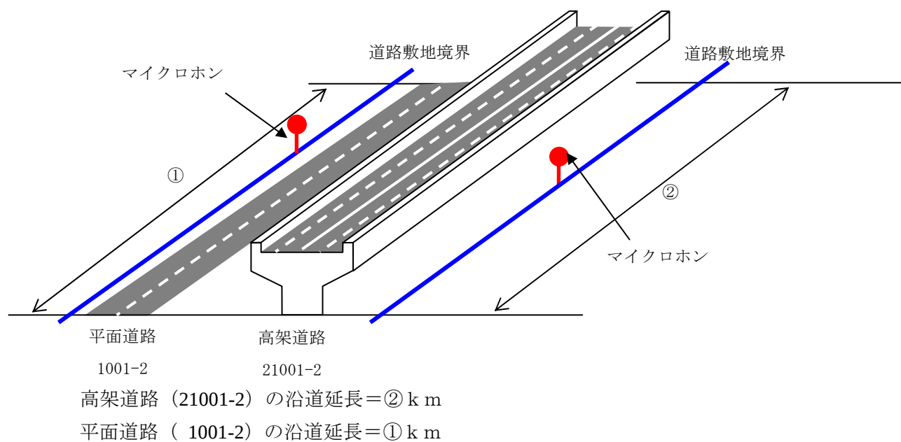
図 5.4.3 騒音を上下方向それぞれ1点で測定している場合の例
