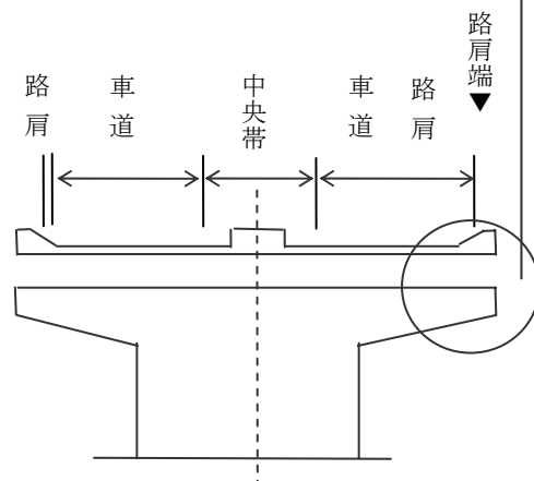
4) 高架構造
