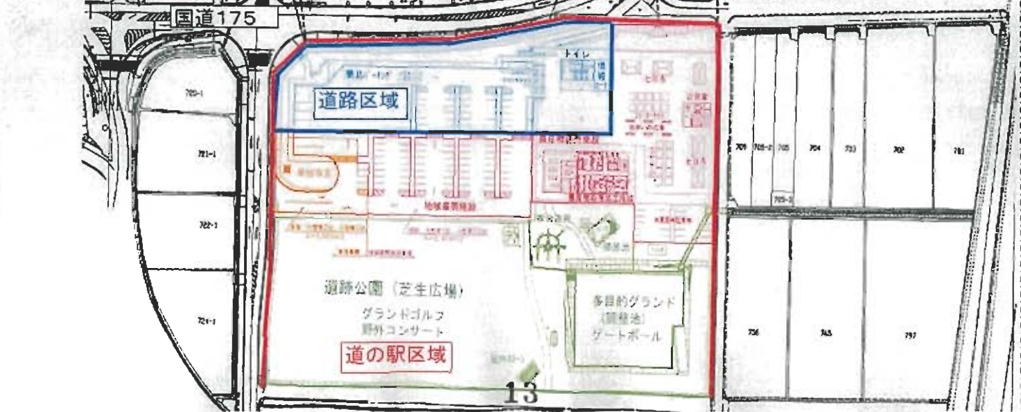
施設配置図(縮尺: 1/2,500 )
