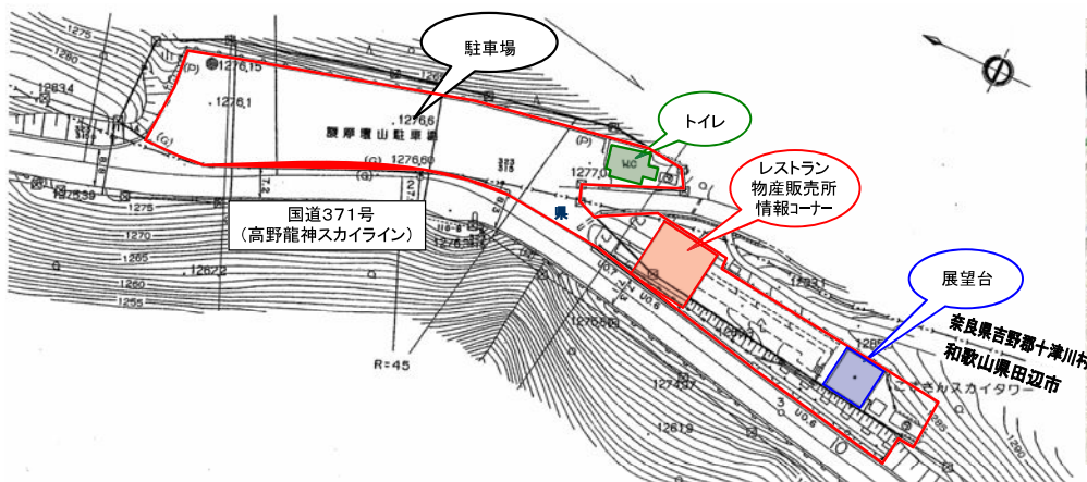
平面図
