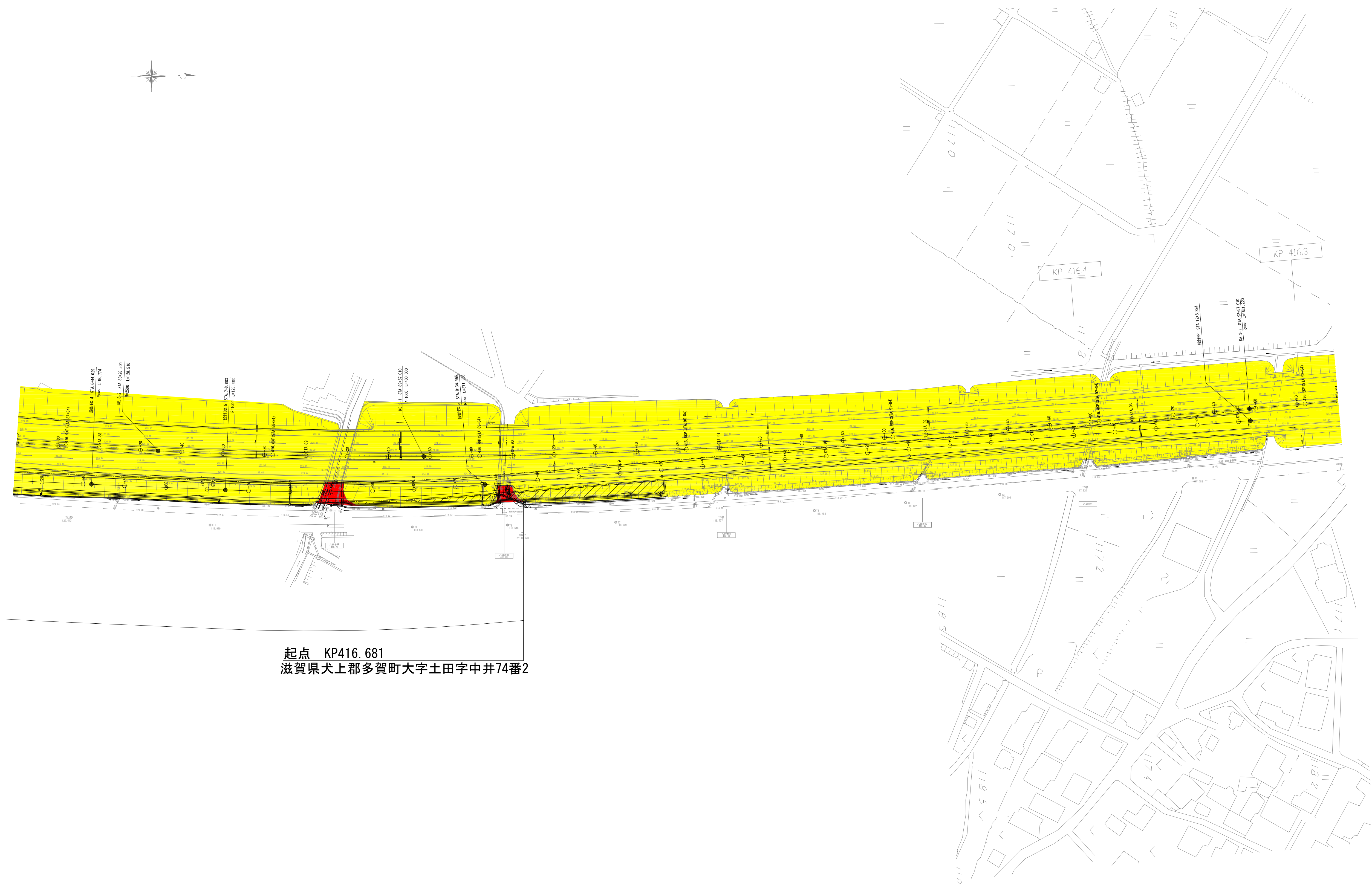
供用開始図(2)
