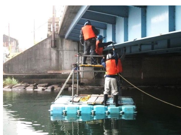
船(フロート)による点検
