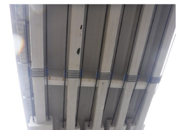
断面修復 外ケーブル補強
