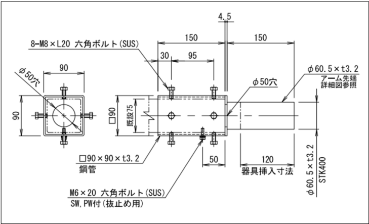
変換アダプタ参考図
