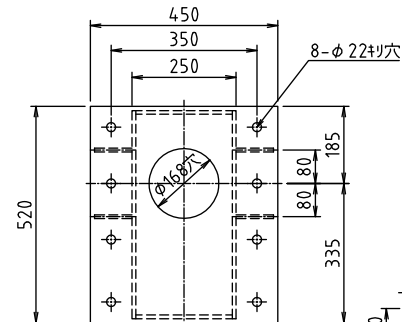
7-Δ側フランジ詳細
