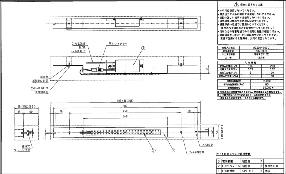
高欄埋込型LEDユニット参考図
