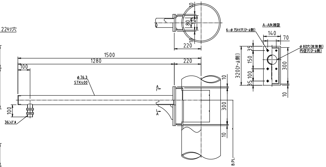
歩行者用信号 フランジ部（参考図）
