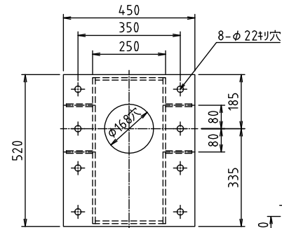
7-Δ側フランジ詳細
