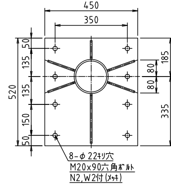
7-Δ側フランジ詳細
