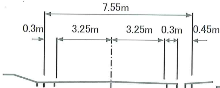
▲国道165号（現道）標準断面図
