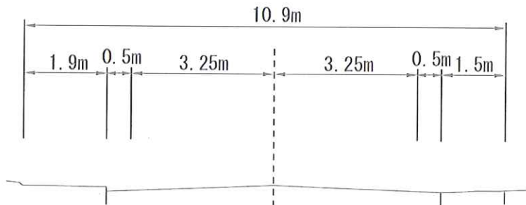
▲国道24号(163号) (現道) 標準断面図
