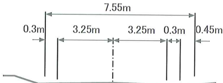
▲国道165号（現道）標準断面図
