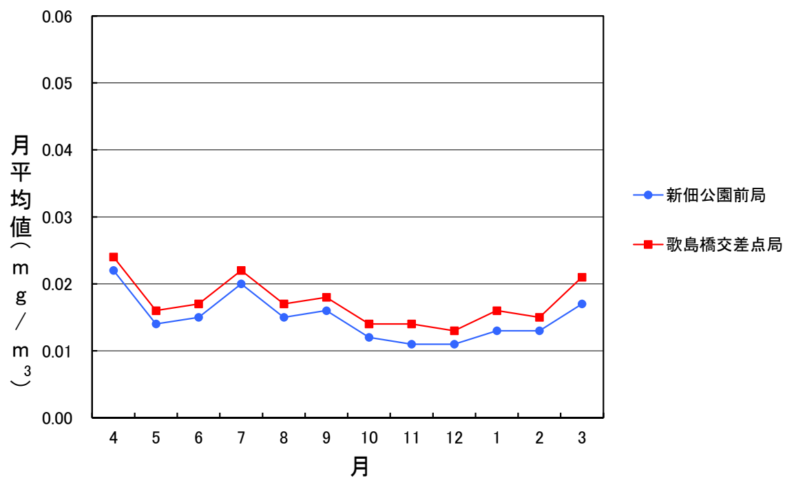
R6年度 浮遊粒子状物質月間値測定結果(大阪2号)
