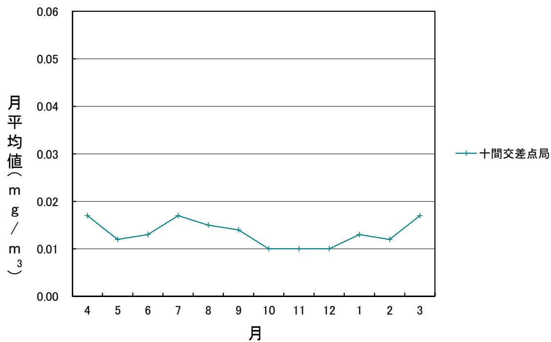
R6年度 浮遊粒子状物質月間値測定結果(兵庫2号)
