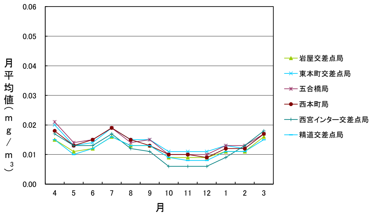
R6年度 浮遊粒子状物質月間値測定結果(兵庫43号)
