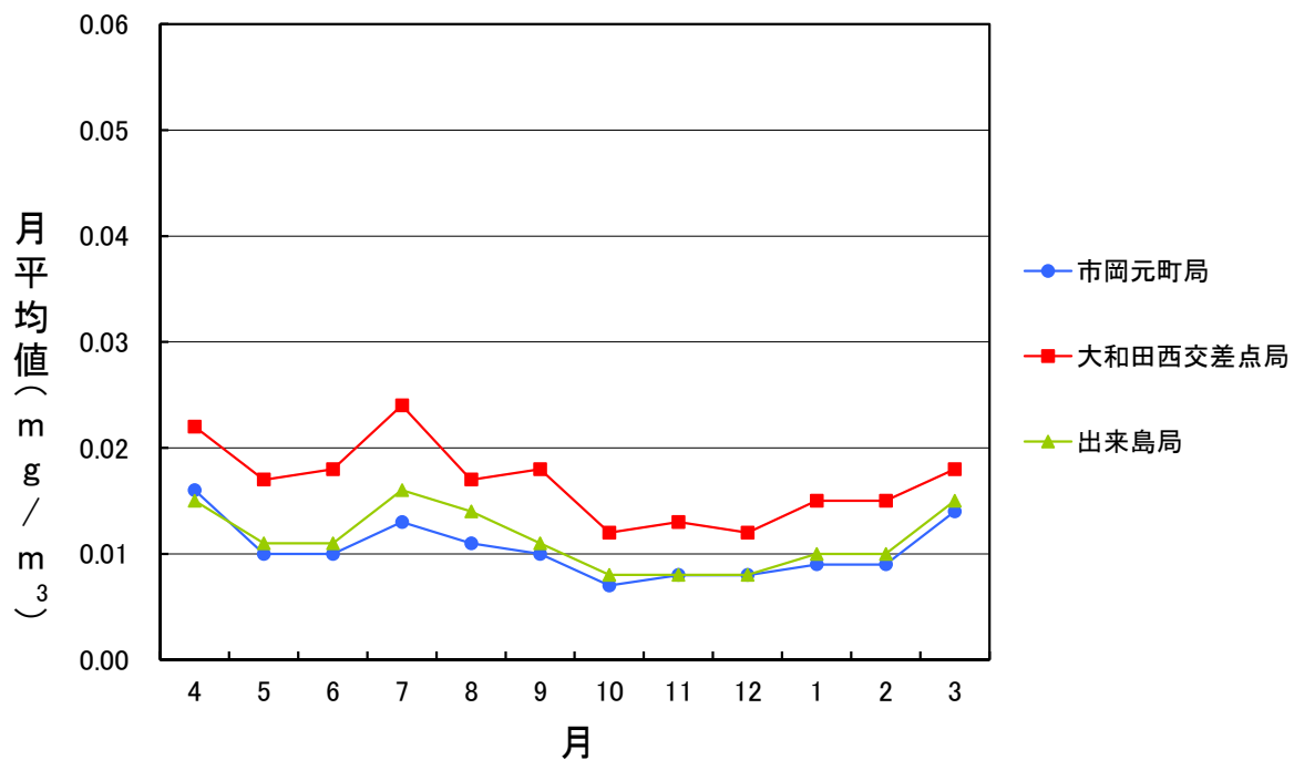
R6年度 浮遊粒子状物質月間値測定結果(大阪43号)
